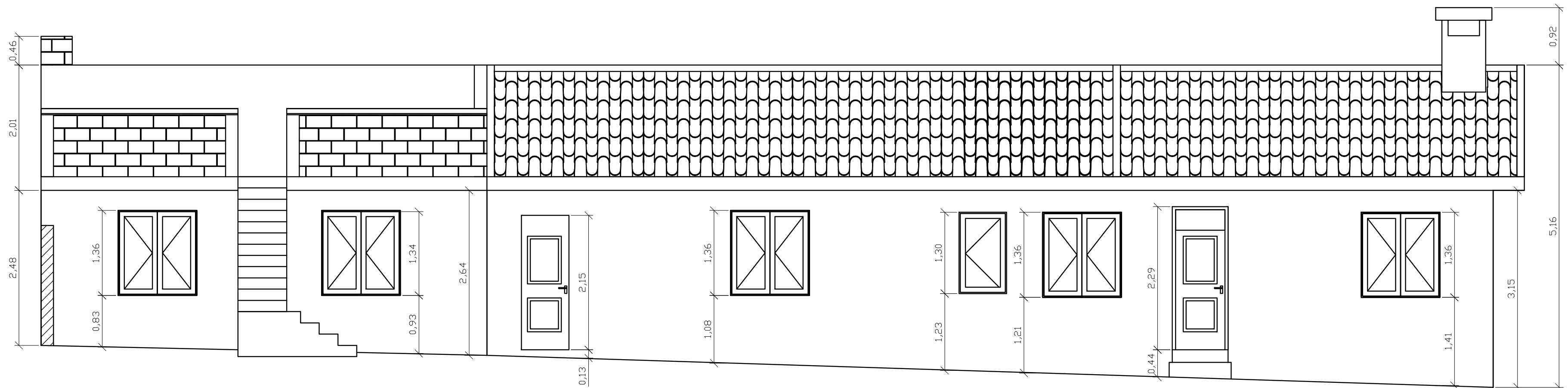
ALZADO OESTE
