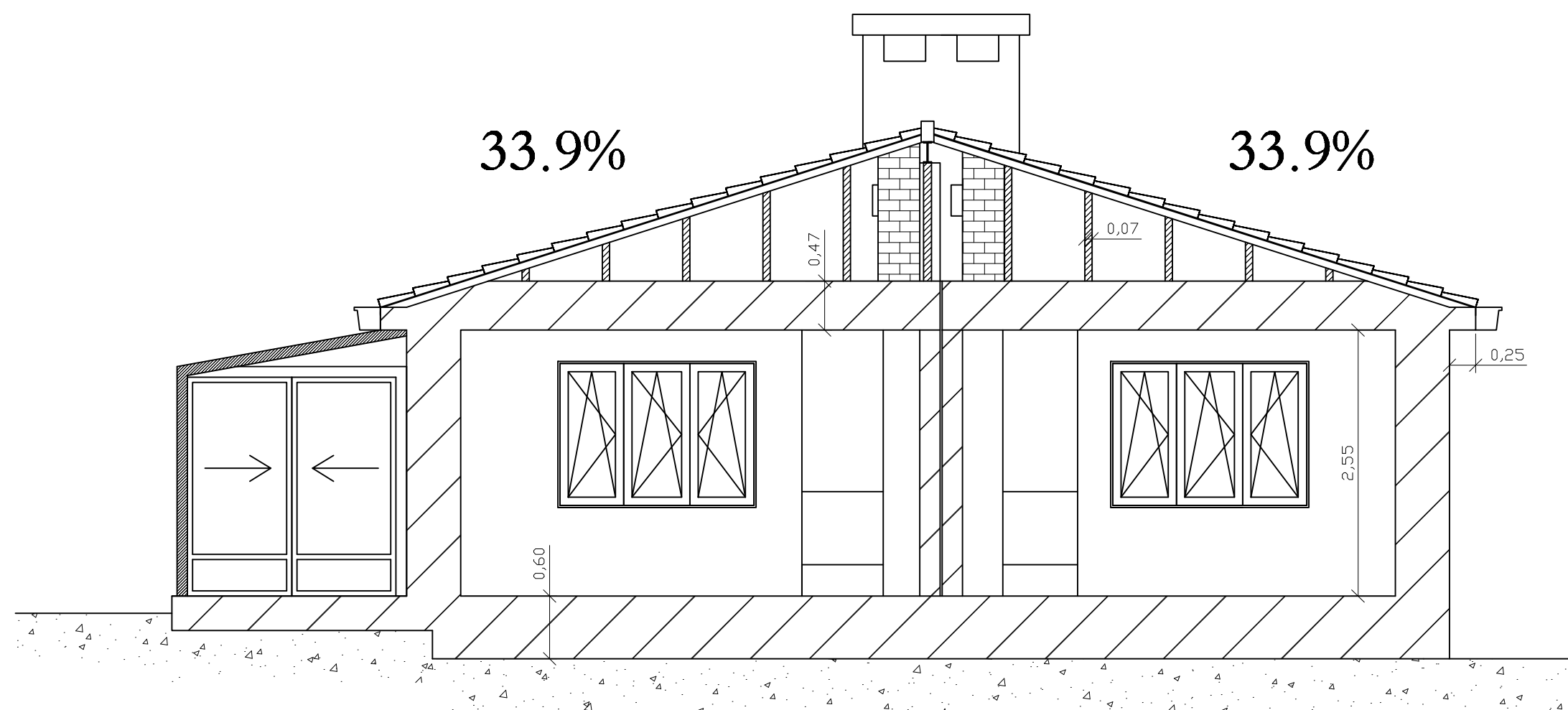
SECCION B-B'
