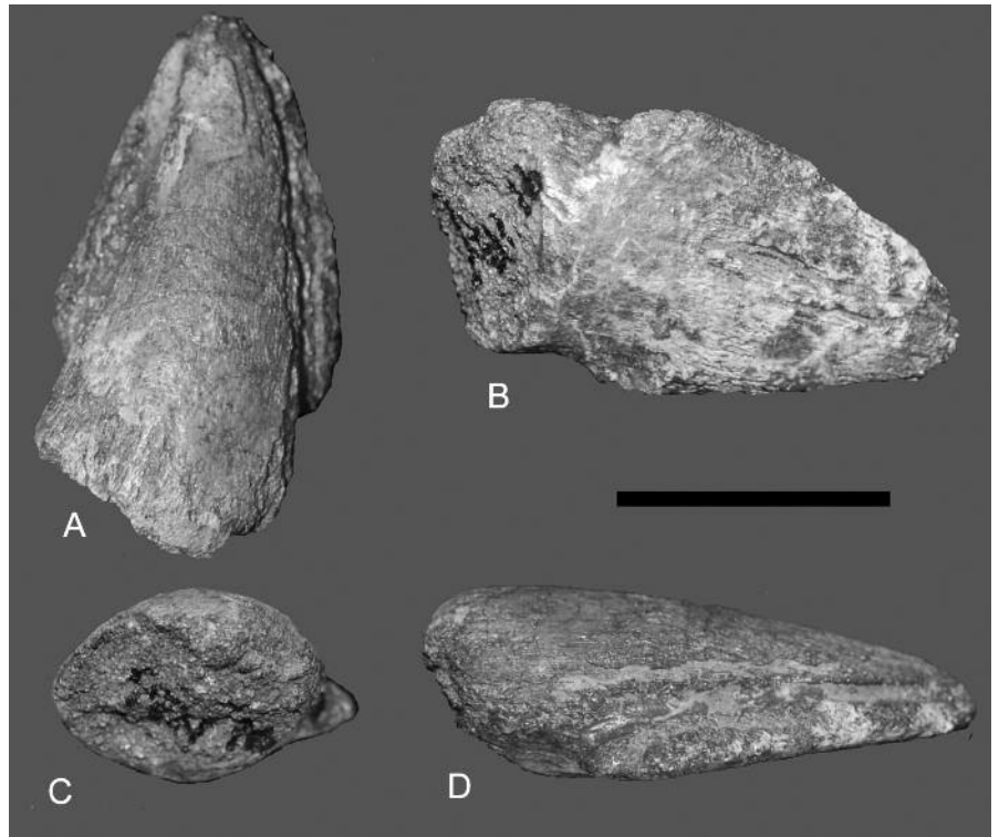
Fig. 2.- Falange ungueal (MOZ-PV:020) de un ornitópodo indeterminado de la Formación Huincul en Agrío del Medio (Neuquén, Patagonia, Argentina). La línea son 20 mm. A: Vista Dorsal. B: Vista plantar. C: Vista proximal. D: Vista lateral.
