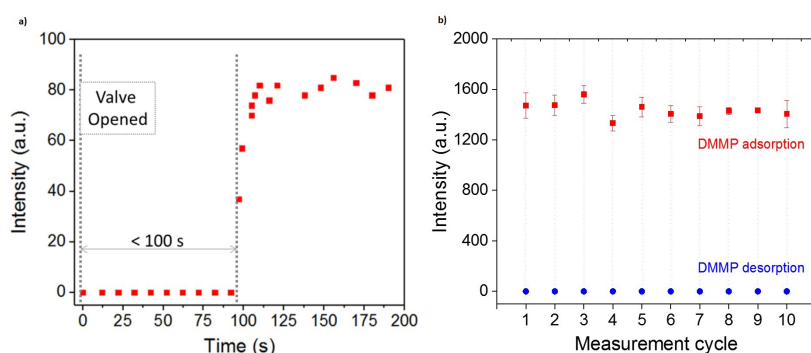
Fig. 6. a) Evolución temporal del pico a 718cm -1 del DMMP sobre AuNP@citrate. Condiciones: 1 mW y 0,5s. b) Evolución del espectro SERS del DMMP cuando se expone el sustrato AuNP@citrate a consecutivos ciclos ON/OFF de DMMP. Condiciones: 1,2 ppmV. (Fuente: Referencia [13]).
