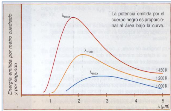
Gráfica del comportamiento del cuerpo negro
