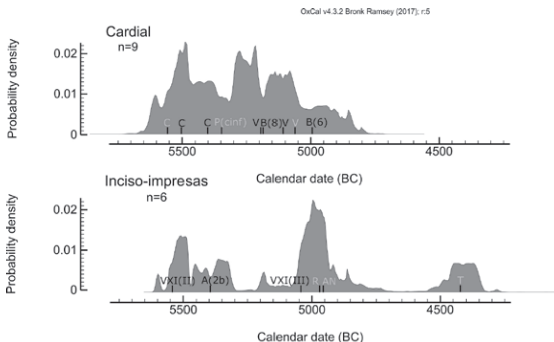
Figura 9. Representación gráfica de las dataciones calibradas del Neolítico antiguo del Bajo Aragón, Maestrazgo y litoral meridional catalán. Se muestran los puntos medios de cada horquilla a 2\sigma . En gris aquellas sobre vida larga. C: Cavet; V: Vidre; B: Botiquería; VXI: Valmayor XI; R: Riols I; AN: Alonso Norte; T: Las Torrazas.
