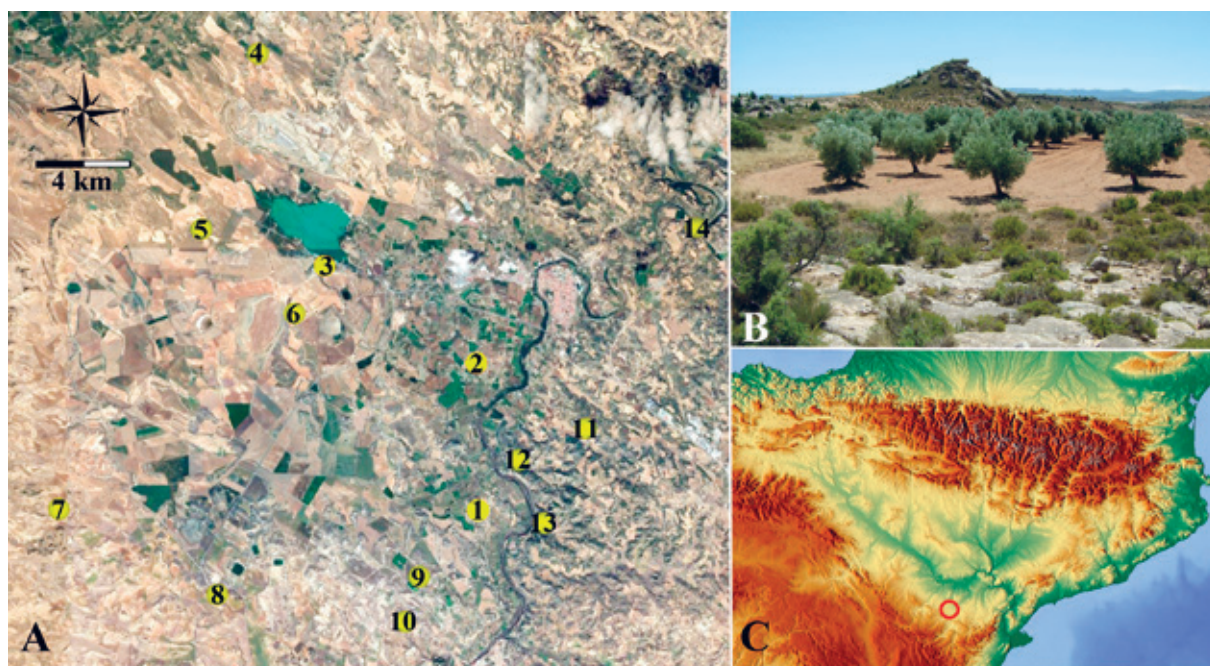
Figura 1. A. Alonso Norte y yacimientos con presencia de Neolítico en el área endorreica de Alcañiz (Google Earth). 1. Alonso Norte; 2. Los Panizales; 3. Las Torrazas; 4. Plaza de Toros de Valdepascual; 5. Las Margaritas; 6. Salada Grande Este I; 7. Acampo Cabañero; 8. Balsa La Salada; 9. Los Pedreñales; 10. Cabezo de Vara I; 11. Pasamán; 12. San Bartolomé; 13. Barranco de La Larga; 14. Torre de Don Mariano B. Vista general de Alonso Norte. C. Situación del grupo de Alcañiz dentro del Valle del Ebro ( https://maps-for-free.com ).
