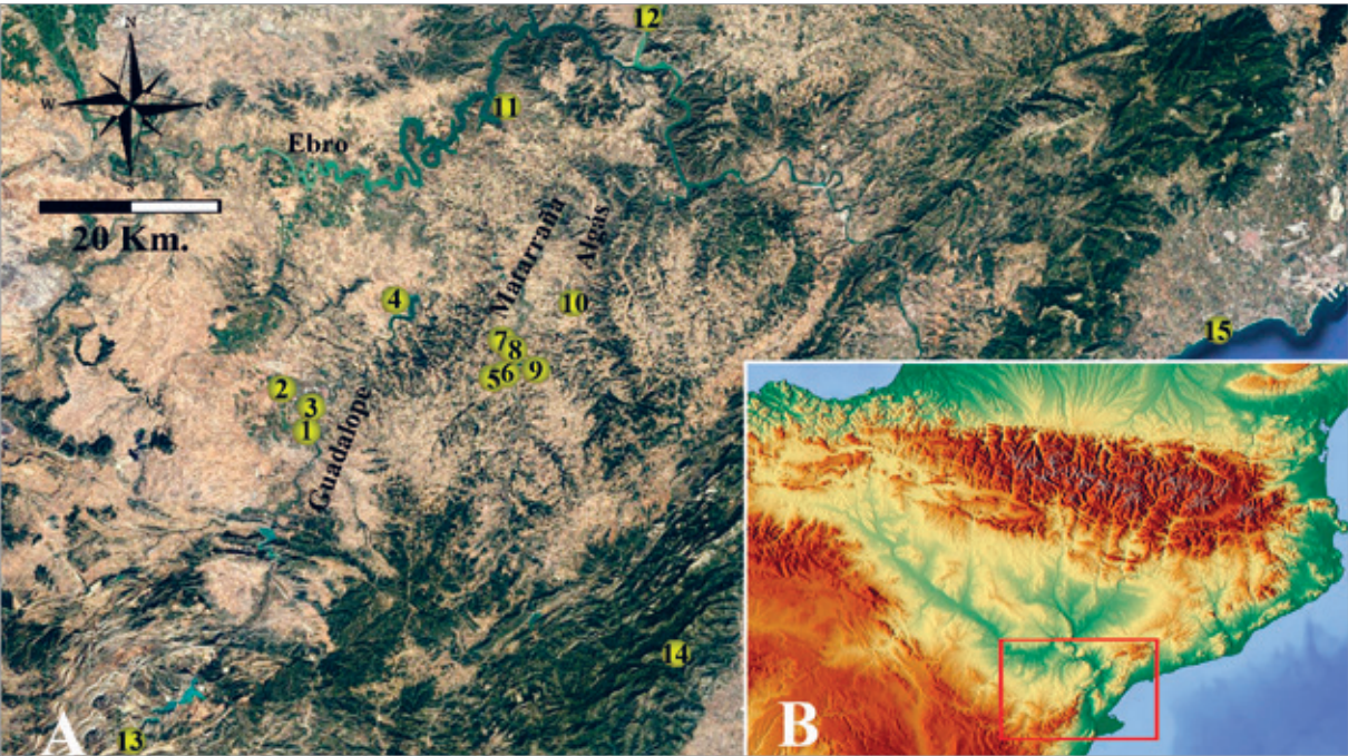
Figura 7. A. Principales yacimientos del Bajo Aragón y zonas próximas. 1. Alonso Norte; 2. Las Torrazas; 3. Los Panizales; 4. Plano del Pulido; 5. Botiquería dels Moros; 6. Secans; 7. Cueva Ahumada; 8. Pontet; 9. Cueva del Llop; 10. Costalena; 11. Valmayor XI; 12. Riols I; 13. Arenal de la Fonseca/Àngel 2; 14. Vidre; 15. El Cavet.
