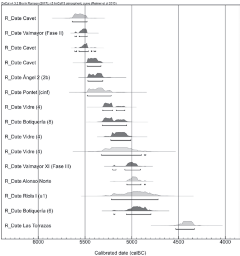
Figura 8. Fechas radiocarbónicas de Alonso Norte y yacimientos del entorno. En gris claro aquellas dataciones realizadas sobre carbón.
