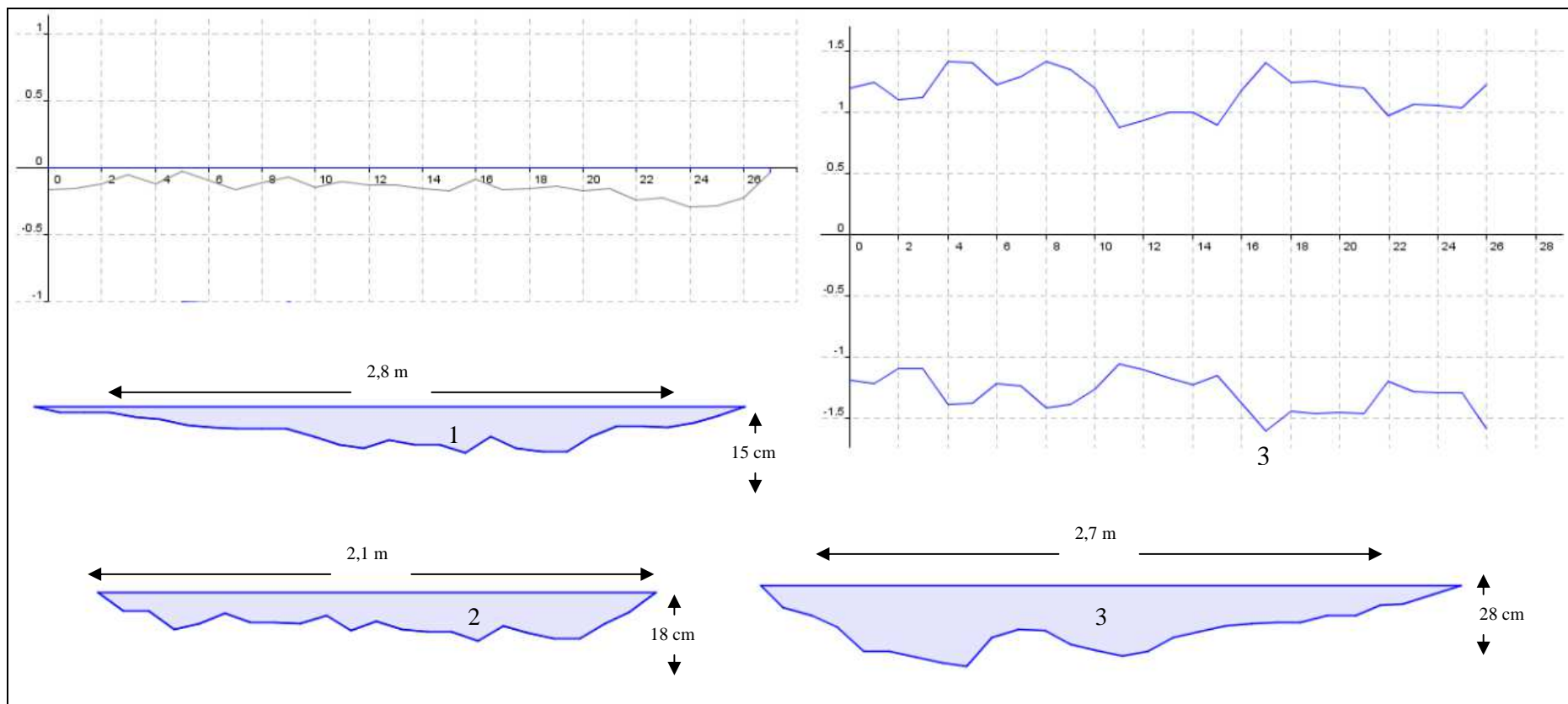
Figura 22: Arriba izquierda: perfil longitudinal del fondo de la estación B; Arriba derecha: Longitud y anchura; Abajo: secciones, longitudes y profundidades de las partes alta, media y baja del tramo.
