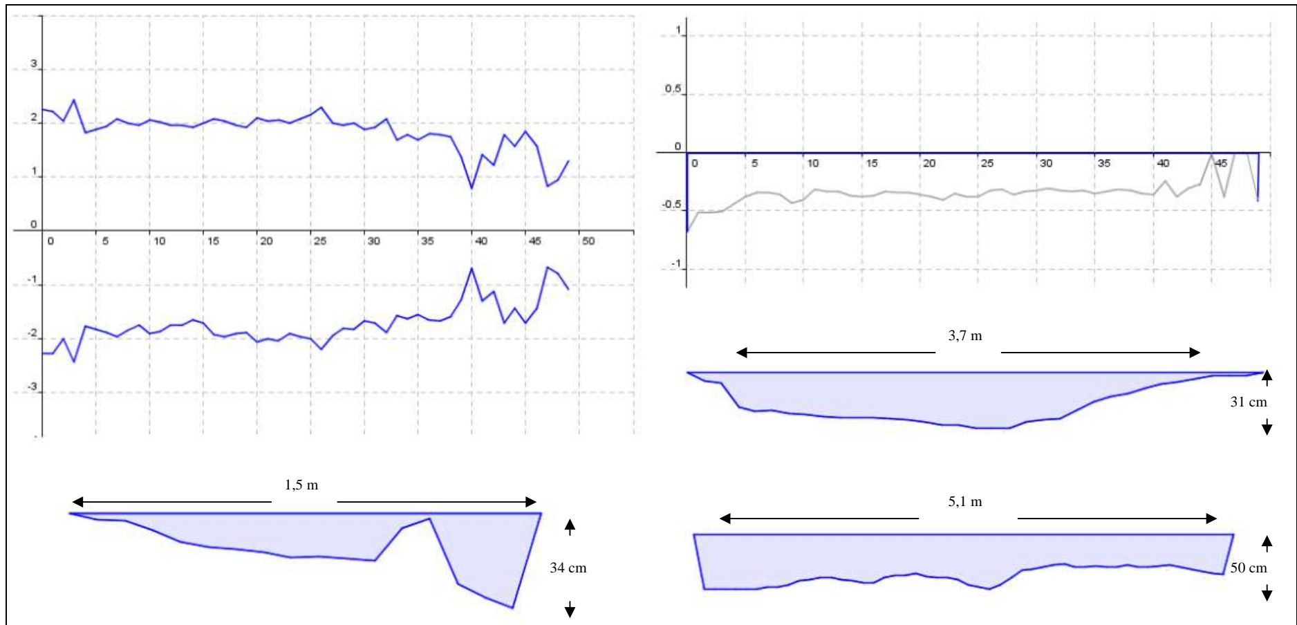
Figura 21: Arriba izquierda: Longitud y anchura de la estación A; Arriba derecha: perfil longitudinal del fondo; Abajo: secciones, longitudes y profundidades de las partes alta, media y baja del tramo.
