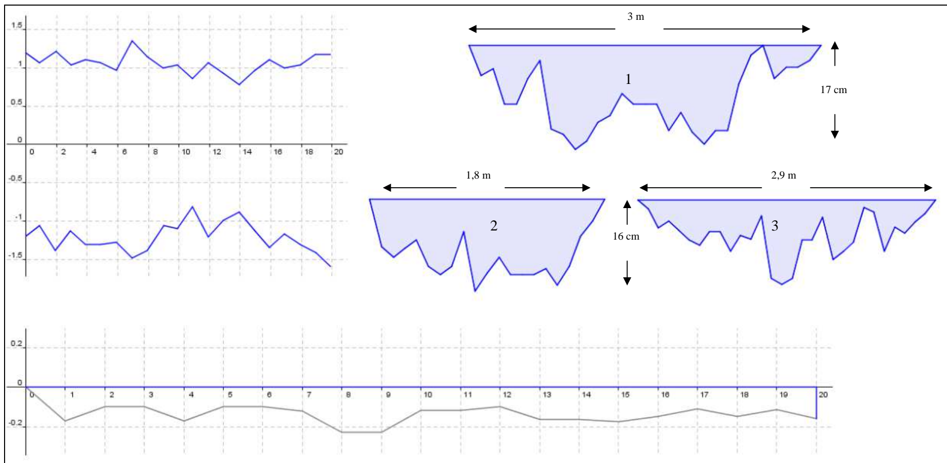
Figura 23: Arriba izquierda: Longitud y anchura de la estación C; Arriba derecha: secciones, longitudes y profundidades de las partes alta, media y baja del tramo; Abajo: perfil longitudinal del fondo.
