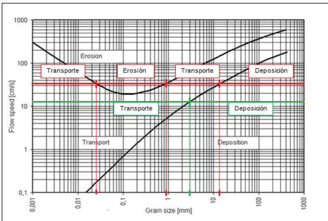
Figura 12: Diagrama de velocidades de flujo en función del diámetro de partícula (Hjulström, 1935). En rojo, resultados obtenidos para la máxima crecida del año 2013. En verde, resultados obtenidos para el caudal base durante el periodo de estudio.
