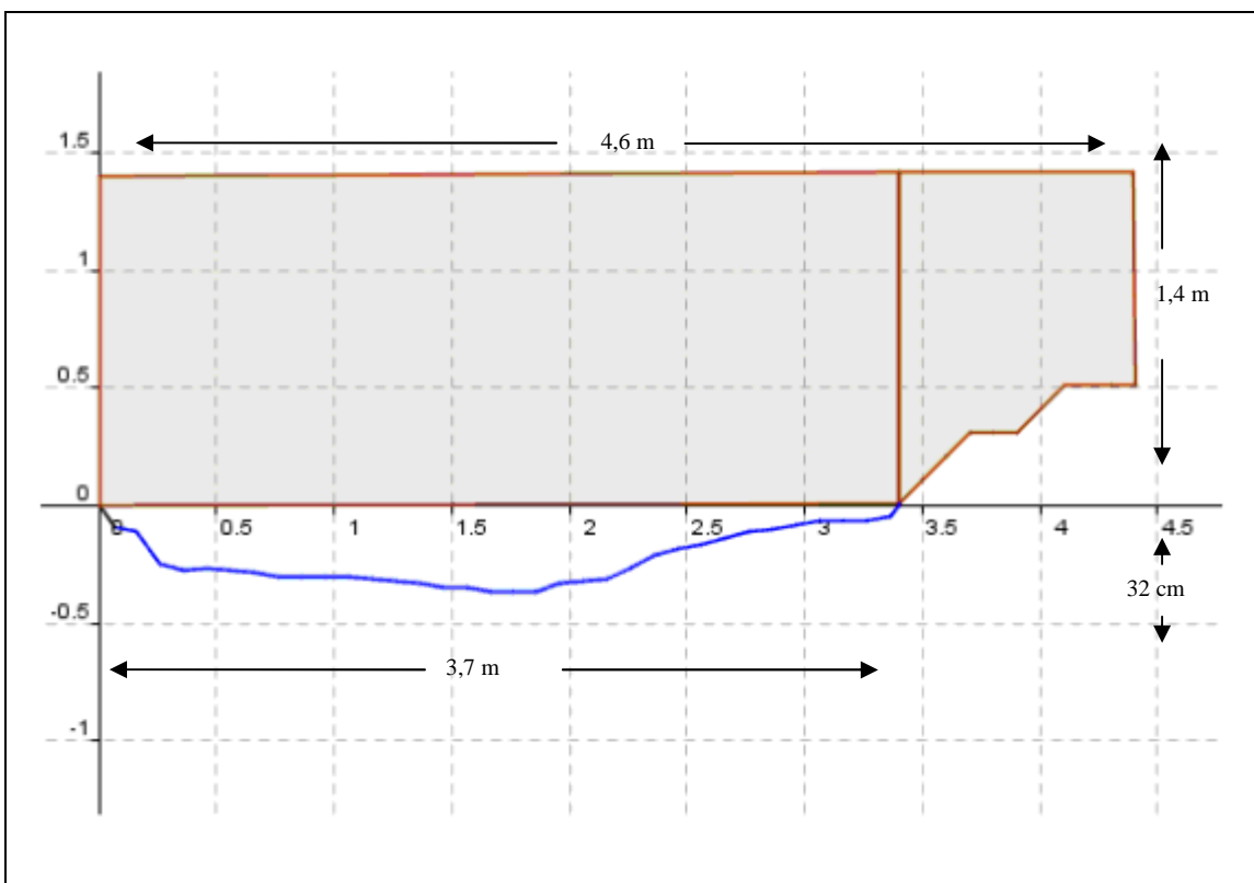
Figura 24: Sección transversal estimada en la estación A para la máxima crecida en 2013. En azul: Sección base del río. En rojo: aumento de la sección durante la crecida.
