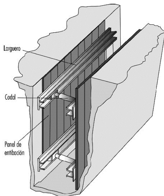
Figura 3. Entubación con tablonera y codales en terrenos granulosos
