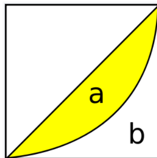
Figura 2.2: Curva de Lorenz
