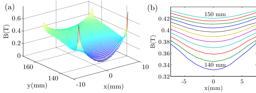
Figura 4.5. Resultados de la simulación del SRM 24/18 en la posición de no alineamiento con i_f=7A : (a) módulo de \mathbf{B} vs. x e y en el polo del estator (las coordenadas en mm x , y de los puntos inferiores y superiores en las aristas del polo son, respectivamente, \pm 7,5 , 132,388 y \pm 7,5 , 162,723 ); (b) módulo de \mathbf{B} vs x en la parte superior del polo a intervalos de y espaciados 10 mm entre 140 y 150 mm
