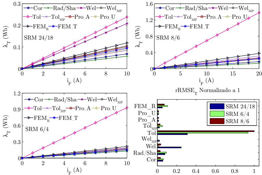
Figura 4.20. Característica flujo concatenado total vs. corriente de fase en la posición de desalineamiento obtenida mediante diferentes procedimientos de cálculo obviando la contribución del material (ver tabla 4.11). rRMSE_T normalizado a la unidad de los procedimientos indicados como Cor, Rad/Sha, Wel, Wel MP , Tol, Tol MP y FEM R considerando FEM T como objetivo.
