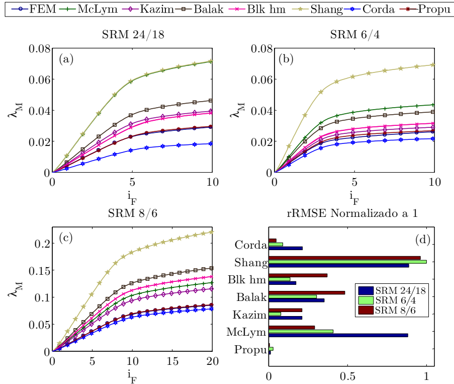
Figura 3.13. (a), (b) y (c) Característica flujo marginal vs. corriente de fase obtenida de la simulación mediante el FEM y diferentes métodos analíticos de cálculo en 2D para los tres motores analizados y (d) representación gráfica de los valores del rRMSE indicados en la tabla 3.3 tras ser normalizados a la unidad.
