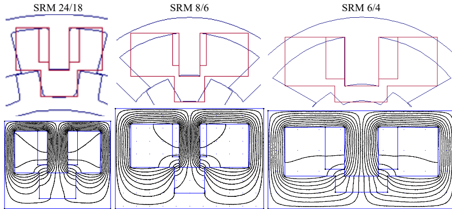
Figura 4.19. Superior: representación rectangular aproximada del entrehierro utilizado para el cálculo de L_{T\_ADEM} y L_{T\_FEM\_R} (color rojo) y geometría exacta empleada para la determinación de L_{T\_FEM} (azul). Inferior: geometría simulada mediante el FEM para la determinación de L_{T\_FEM\_R} .
