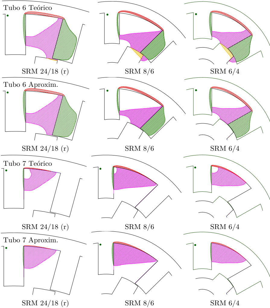
Figura 4.8. Detalle de los tubos 6 y 7 en los tres motores bajo estudio. Se muestra el recorrido teórico y su aproximación (imágenes vectoriales).
