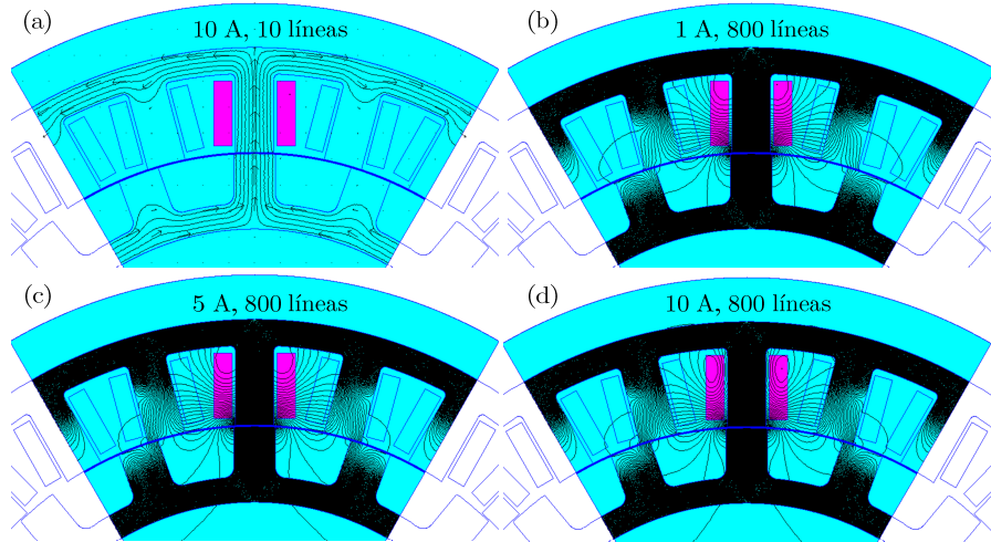
Figura 3.2. Representación en 2D por el programa FEMM de las líneas de flujo (trayectorias equipotenciales del potencial magnético vector \mathbf{A} ) en el prototipo del SRM en la posición de alineamiento: (a) con i_F=10 A y solo 10 líneas; (b), (c) y (d) con i_F=1, 5 y 10 A y 800 líneas, respectivamente (el flujo se dispersa en el polo del estator y se ensancha en el entrehierro). Los rectángulos rosas representan la corriente en la bobina excitada y las flechas en (a) el sentido y la dirección de \mathbf{B} .
