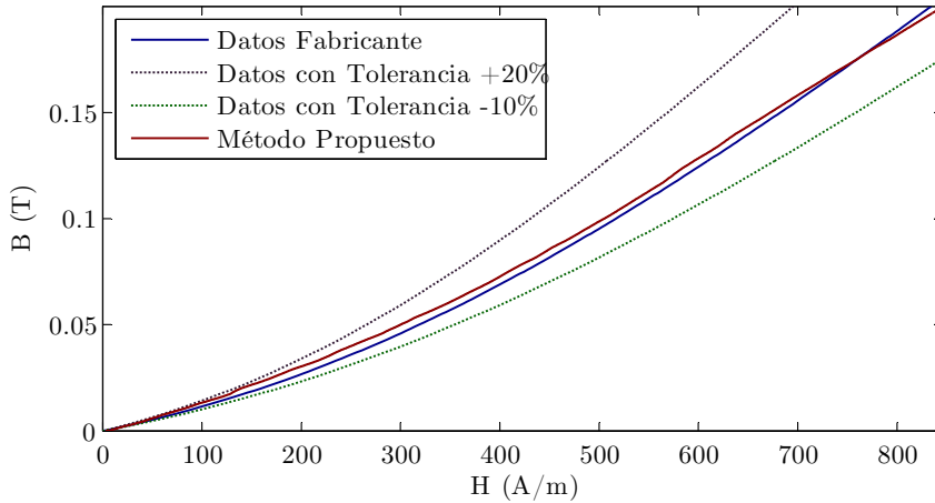
Figura 2.7. Curvas de primera imanación en la región de Rayleigh obtenidas con los datos proporcionados por el fabricante y por el método propuesto.
