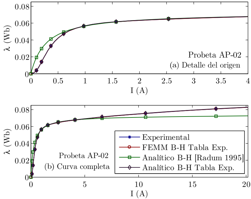
Figura 2.12. Relación entre el flujo concatenado y la corriente en la probeta P-AP02 obtenida experimentalmente, mediante FEMM con los valores B - H experimentales, analíticamente según (2.24) y analíticamente según (2.12) con \mu = B/H obtenida de los valores experimentales. (a) Detalle hasta 4 A; (b) rango completo.
