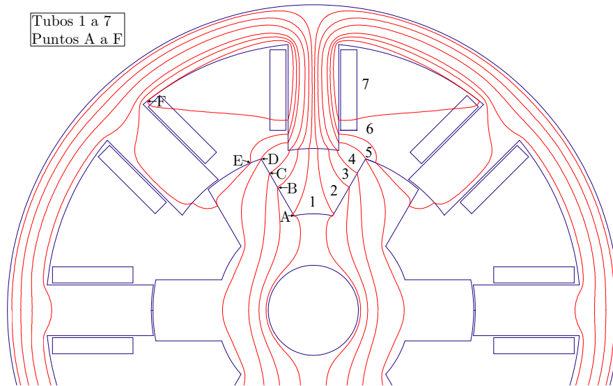
Figura 4.3. Representación gráfica de las líneas equipotenciales de \mathbf{A} que limitan los 7 tubos de flujo (imagen vectorial).
