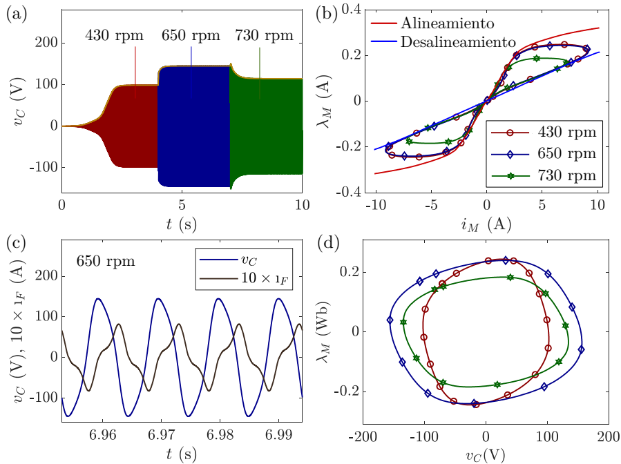
Figura 6.23. Izqda: Simulación a tres velocidades: por debajo de la velocidad nominal (430 rpm, 164 \mu\text{F} ), a la velocidad nominal (650 rpm, 72 \mu\text{F} ) y por encima de la velocidad nominal (730 rpm, 57 \mu\text{F} ). a) Tensión en el condensador y su envolvente superior (marrón); c) Estado estacionario de la corriente de fase y la tensión en el condensador a la velocidad nominal. Dcha.: b) Trayectorias en el sentido de las agujas del reloj para las mismas velocidades, cuyas áreas escaneadas representan la energía transformada por ciclo (hasta la velocidad nominal, la energía por ciclo es similar, por encima de ella el área cerrada es más pequeña); d) Ciclo límite correspondiente a tres velocidades (hasta la velocidad nominal (650 rpm), el pico del flujo concatenado de magnetización está en un máximo y permanece casi constante).
