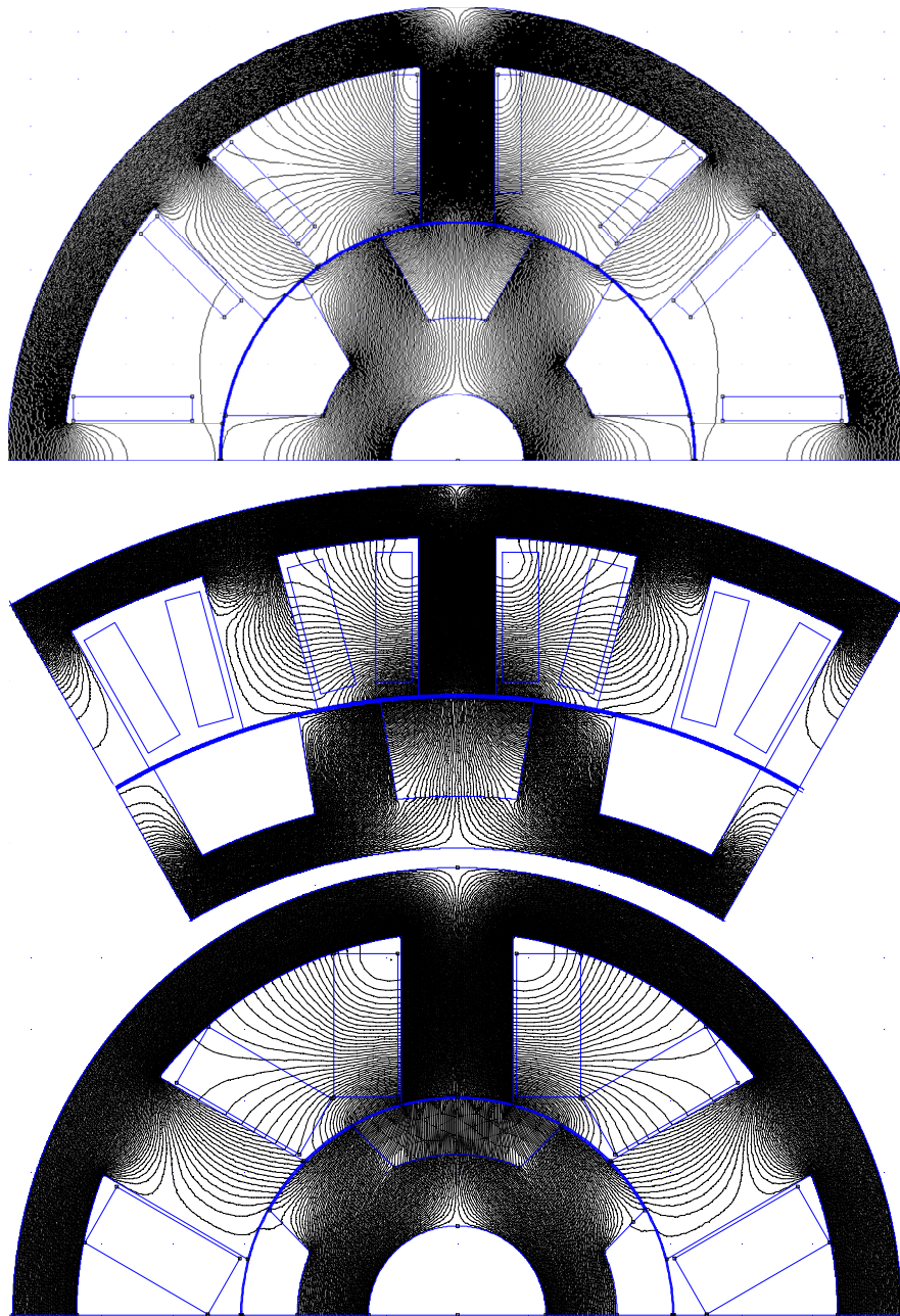
Figura 4.2. Resultados de la simulación del SRM 8/6 ( i_F = 14 A), el SRM 24/18 ( i_F = 7 A) y el SRM 6/4 ( i_F = 7 A) en la posición de no alineamiento, mostrando 260 líneas equipotenciales de \mathbf{A} (imágenes vectoriales ampliables sin pérdida de resolución en el documento en formato digital).
