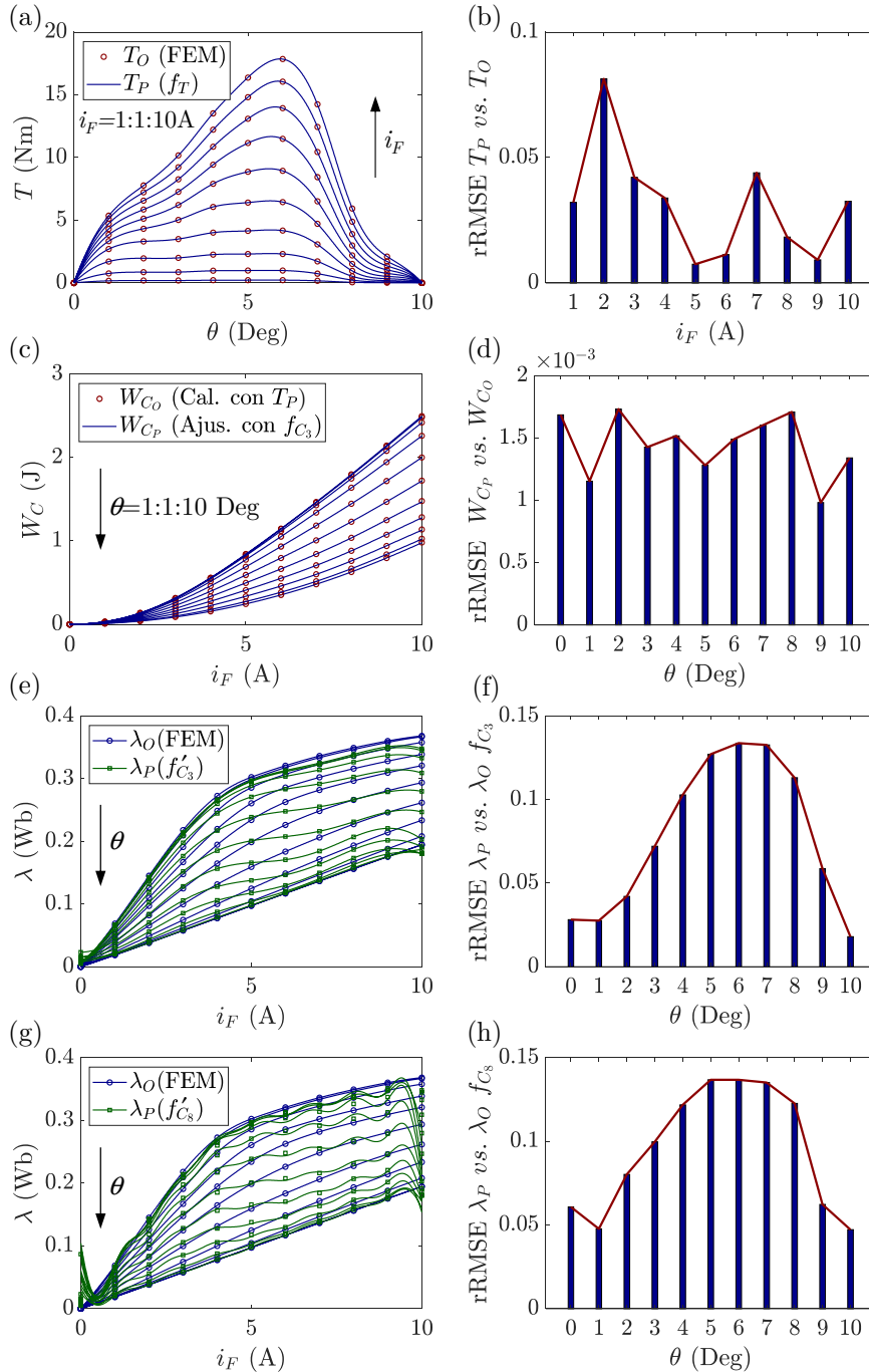
Figura 5.7. Resultado de la determinación de la coenergía ( c ) y el flujo concatenado ( e y g ) a partir del par (a). Error rRMSE entre los valores objetivo (O) y calculados (P) analíticamente del par (b), la coenergía (d) y el flujo concatenado (f y h).
