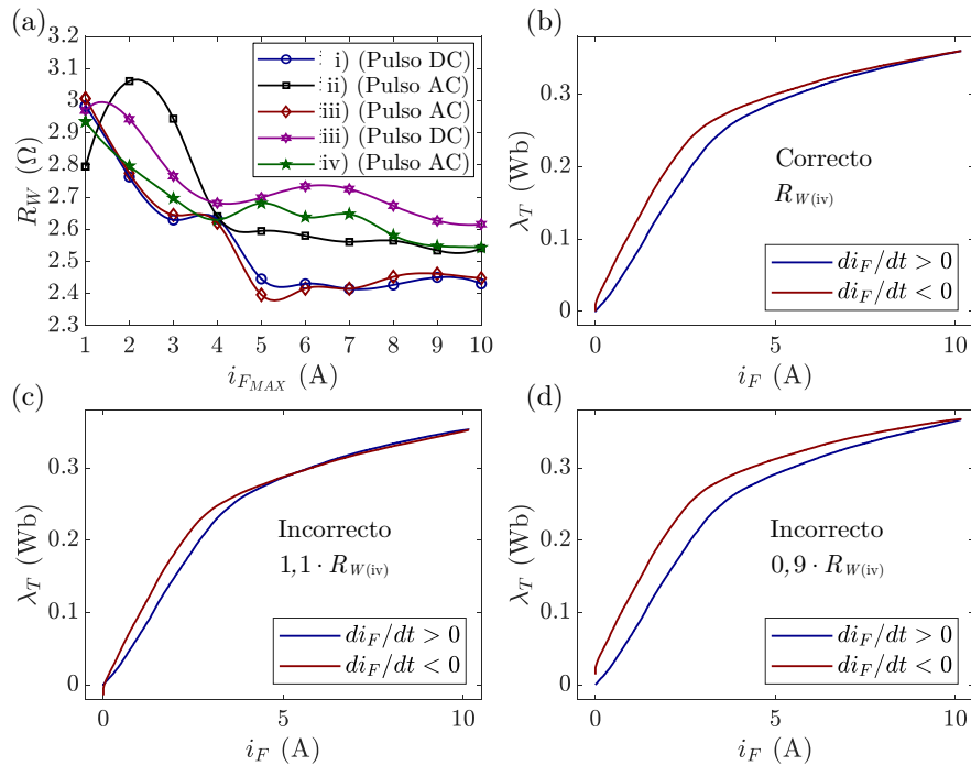
Figura 6.10. Relación en la posición de alineamiento entre la resistencia del devanado R_W y el valor máximo de la corriente de fase i_{FMAX} determinada mediante los 4 procedimientos, para i_{FMAX} entre 1 y 10 A con incrementos de 1 A (a); relación \lambda_T vs. i_F en la posición de alineamiento habiendo obtenido R_W mediante el procedimiento (iv) (b) y en el caso de modificar el valor de R_W un 10% (c) y un -10% (d).
