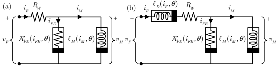
Figura 6.7. Circuitos equivalentes de una fase en un SRM con el rotor bloqueado: (a) considerando la saturación y las pérdidas en el material, pero despreciando el flujo de dispersión; (b) considerando además el flujo de dispersión.
