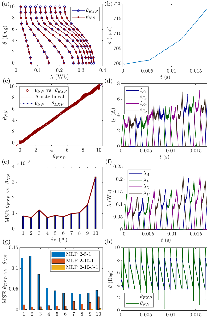
Figura 6.3. Relación \theta vs. \lambda tomando como parámetro i_F (a); correlación entre los valores de la posición experimental \theta_{EXP} y los obtenidos del MLP 2-10-5-1 \theta_{NN} (c); MSE entre los valores \theta_{EXP} y \theta_{NN} en las estructuras 2-10-5-1, 2-10-1 y 2-5-1 (e y g); velocidad angular del motor en rpm (b), corrientes (d) y flujos concatenados (f) en cada fase y \theta_{EXP} y \theta_{NN} a la salida del MLP 2-10-5-1 (h).
