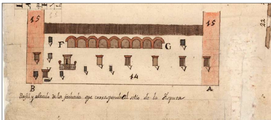
Fig. 49. Perfil y alzado de la fachada posterior del palacio de los condes de Gómara, por Miguel Antonio de Olasagarre, 1774. AGN.
