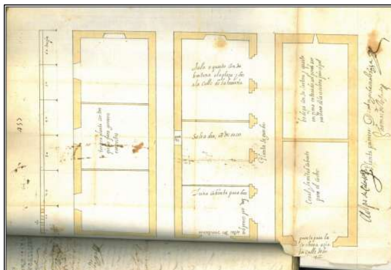
Fig. 92. Trazo para la construcción de un cuarto de casa para la vivienda de José de La Peña en Valtierra. 1666. AHPLR.
