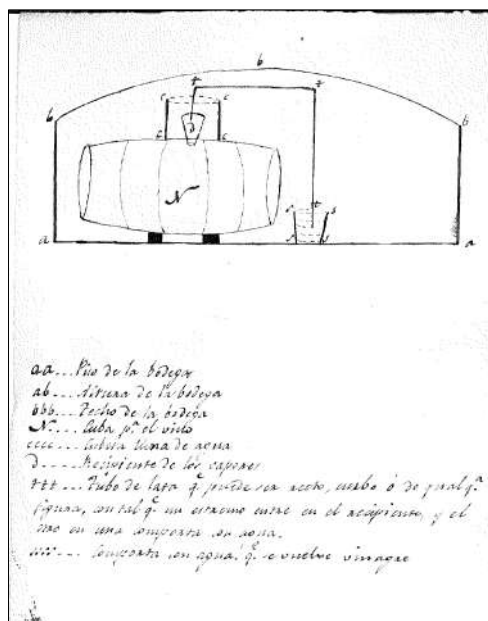
Fig. 31. Dibujo para la instalación de una cuba para vino en la bodega. ACR.
