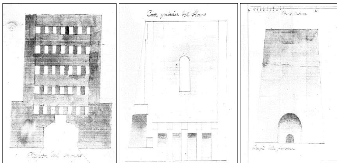
Fig. 28. Planos de la nueva tejería por Ignacio Asensio. 1797. APT.
