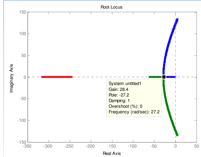
Fig. 5. Lugar de las raíces de la compuerta.
