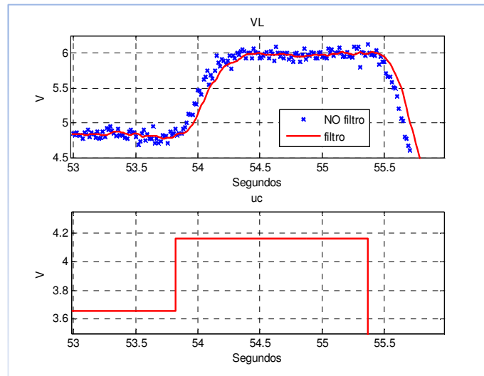
Fig. 9. Implementación del ensayo Ziegler-Nichols en bucle abierto.
