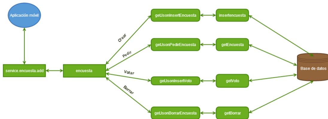
Figura 4.1 Diagrama de bloques del funcionamiento del servidor.
