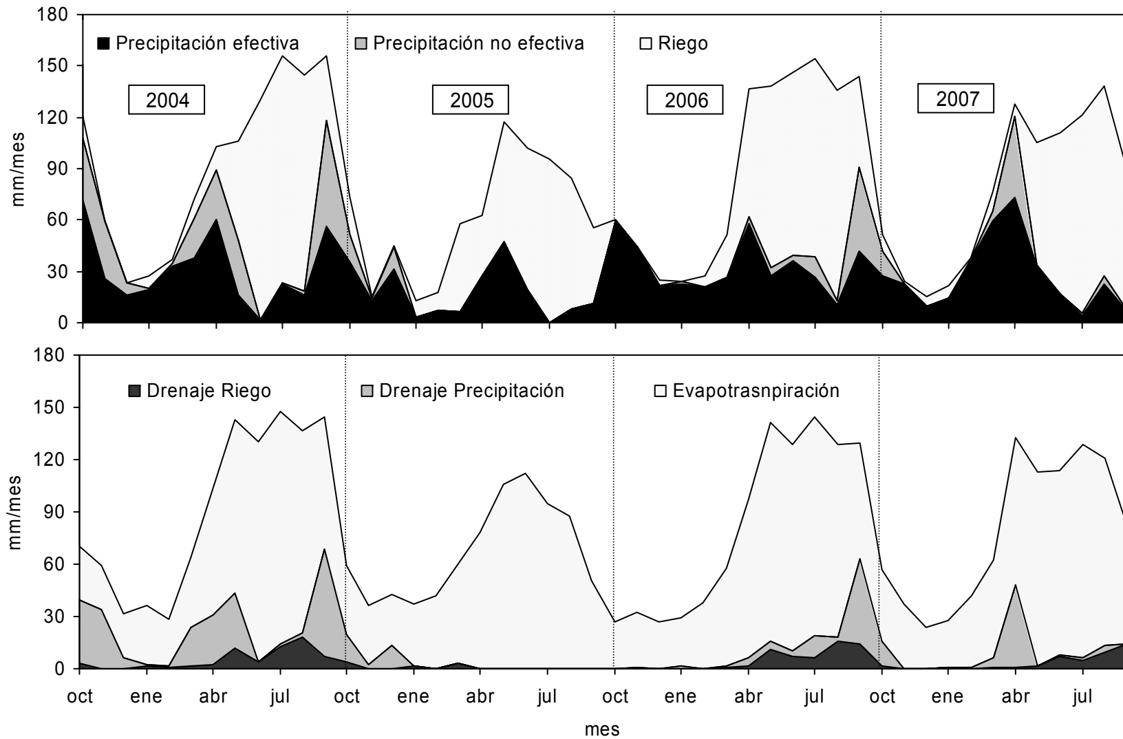
Fig. 4.3. Evolución mensual de las entradas (riego, precipitación efectiva y no efectiva) y salidas (evapotranspiración y drenaje de la precipitación y riego) obtenida del balance de agua en el suelo durante los cuatro años de estudio (2004-2007).
