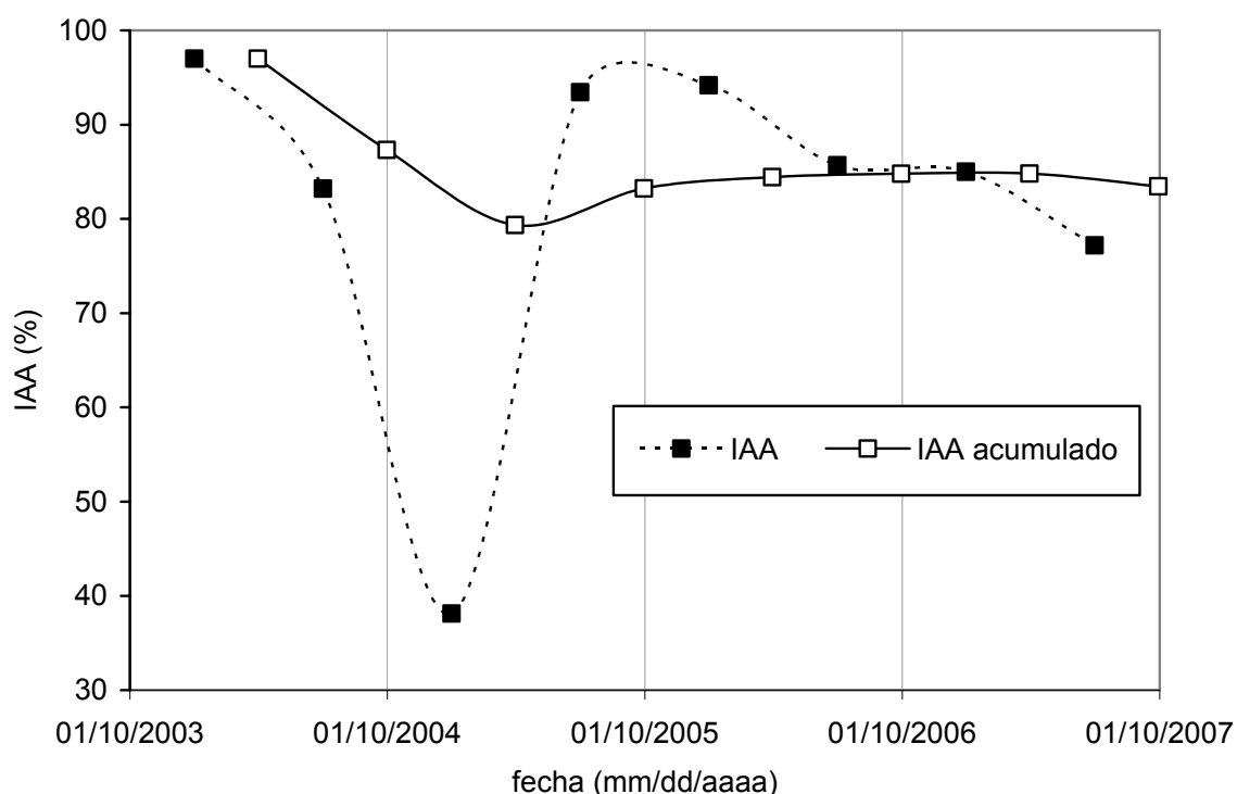
Fig. 4.5. Evolución semestral del Índice de Aprovechamiento de Agua (IAA) para el conjunto del sistema evaluado en los cuatro años de estudio (2004-2007).
