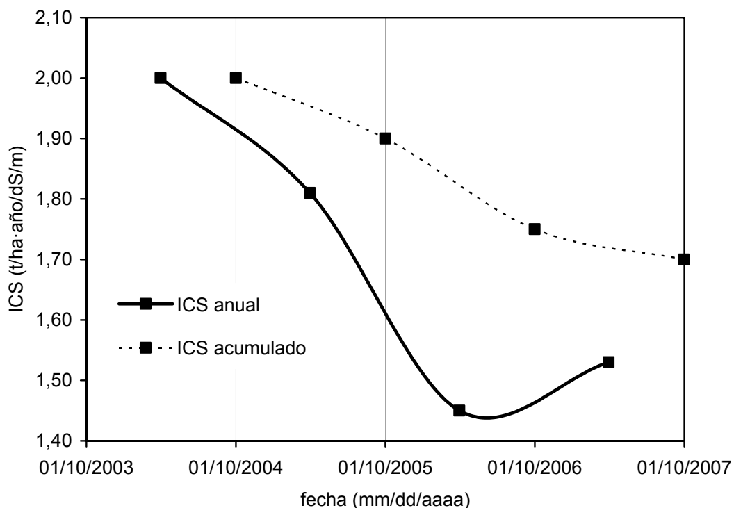
Fig. 5.2. Índice de Contaminación por Sales (ICS) del área regable incluida en la cuenca del Arba en los cuatro años de estudio (2004-2007) y anualmente acumulado.
