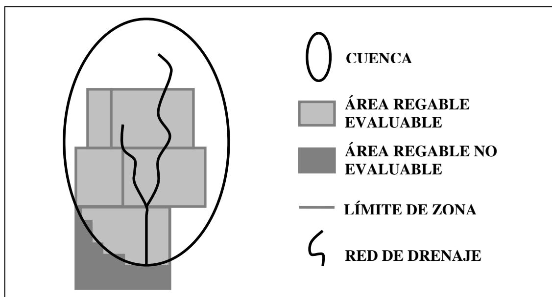
Fig. 3.1. Croquis de una hipotética cuenca en la que el área regable a evaluar se reparte en cinco “zonas”, de las cuales parte de una de ellas se localiza en el exterior de la cuenca y por tanto no es evaluable en el proyecto.
