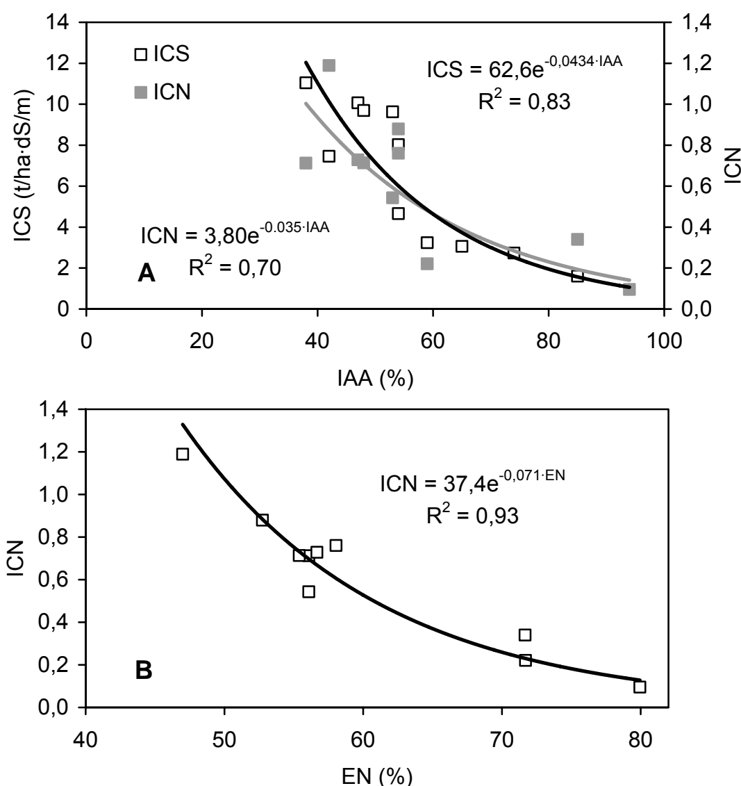
Fig. 3.2. A- Relaciones entre el Índice de Aprovechamiento del Agua (IAA) y los Índices de Contaminación Salina (ICS) y por Nitratos (ICN). B- Relación entre la Eficiencia de aplicación de Nitrógeno (EN) y el Índice de Contaminación por Nitrato (ICN).
