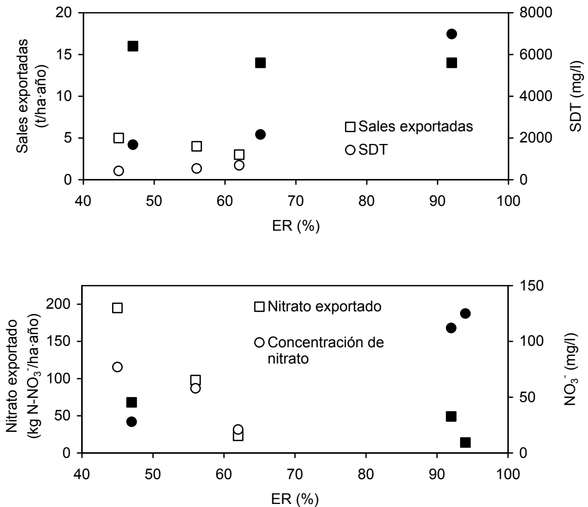
Fig. 2.2. Relación entre la eficiencia de riego y las concentraciones y masas de sales y nitratos exportadas en siete regadíos estudiados de la cuenca del Ebro. Los símbolos sólidos se corresponden a los regadíos yesíferos y salinos.
