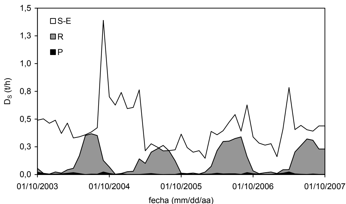
Fig. 5.1. Evolución mensual de las sales exportadas en el drenaje propio del sistema evaluado ( D_s ) y la contribución a éste de las sales introducidas con la precipitación (P), riego (R), y disolución de materiales geológicos (S-E).
