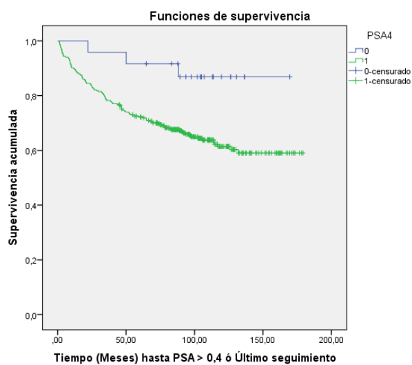
Figura 4.18: Curvas de supervivencia.PSA4
