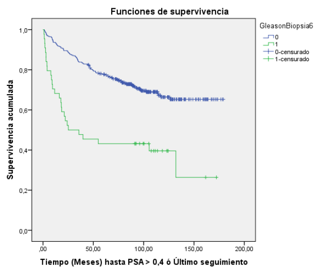
Figura 4.19: Curvas de supervivencia.GleasonBiopsia6
