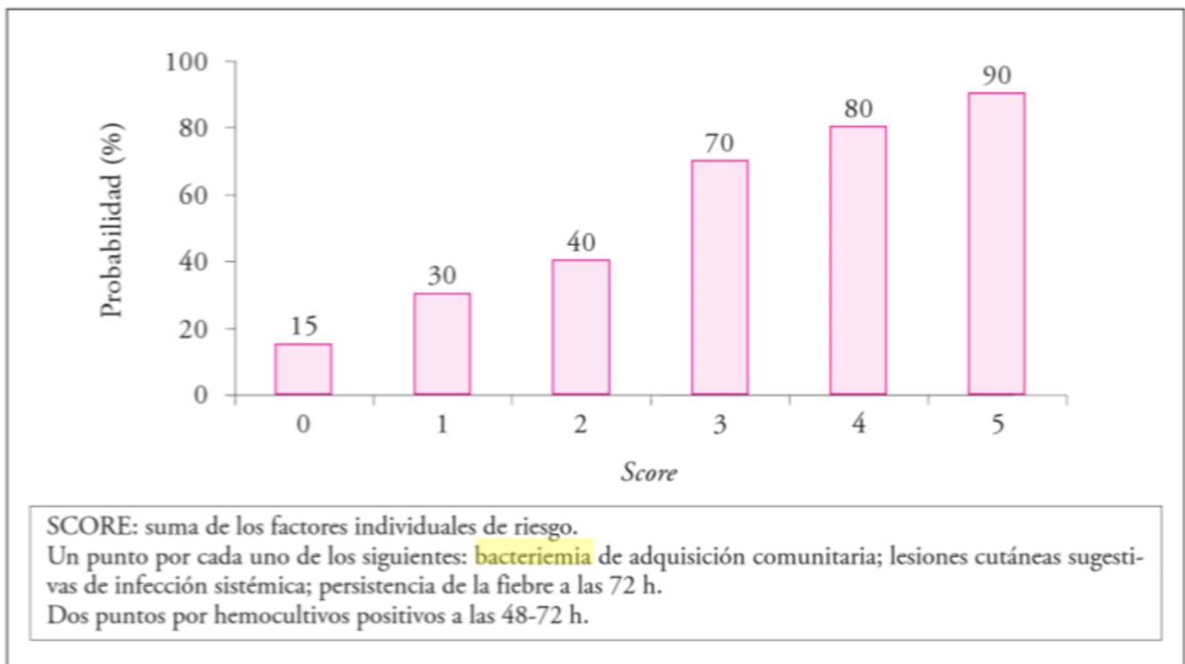
Figura 3: SCORE complicaciones.
