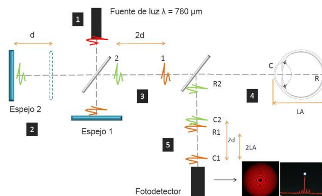
Fig.18. Esquema del funcionamiento del biómetro óptico.
