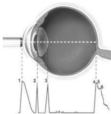
Fig.17. Esquema de los ecos obtenidos mediante el método de biometría ultrasónica de contacto.
