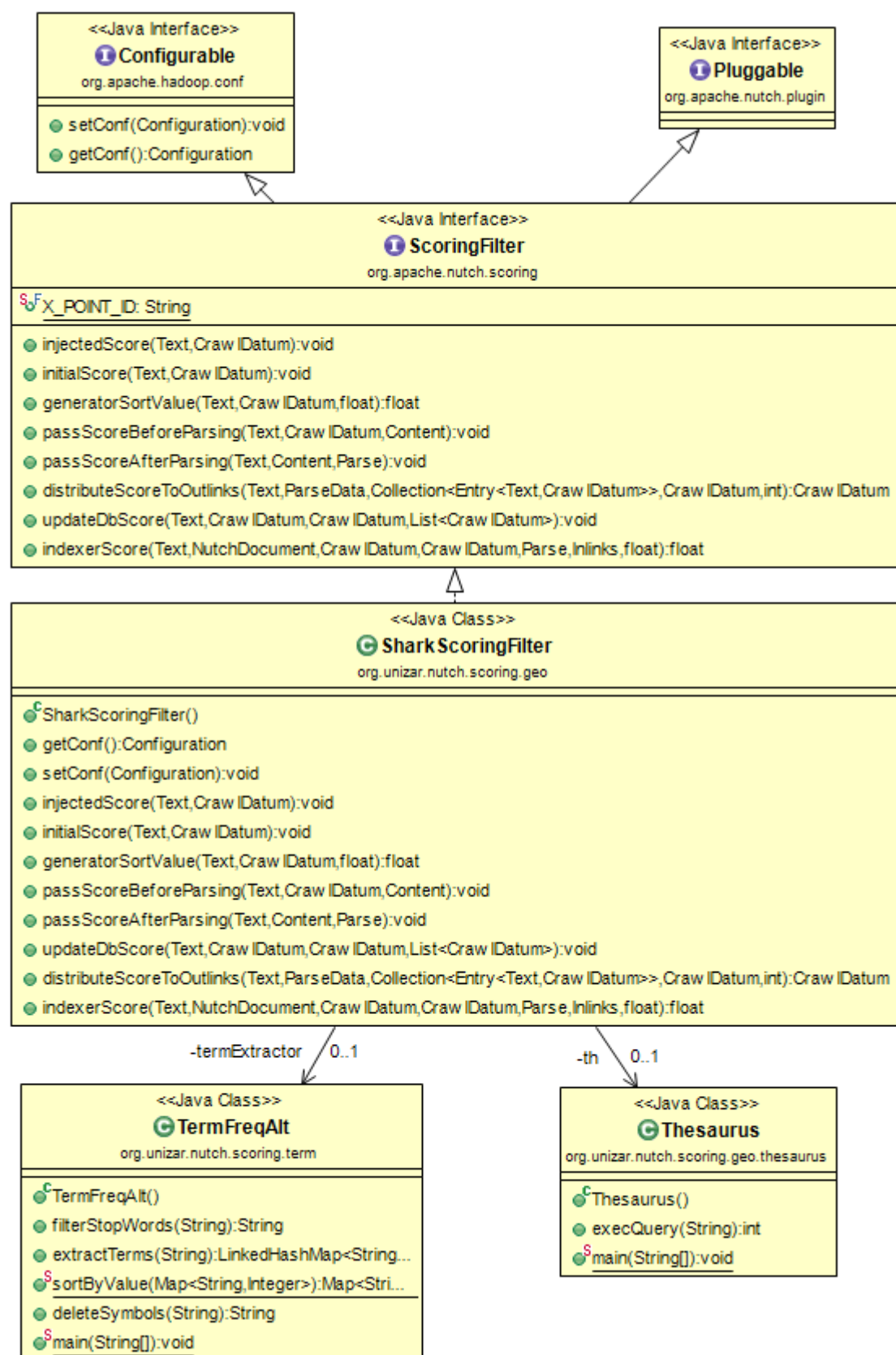
Figura 8: Diagrama de clases de SharkScoringFilter
