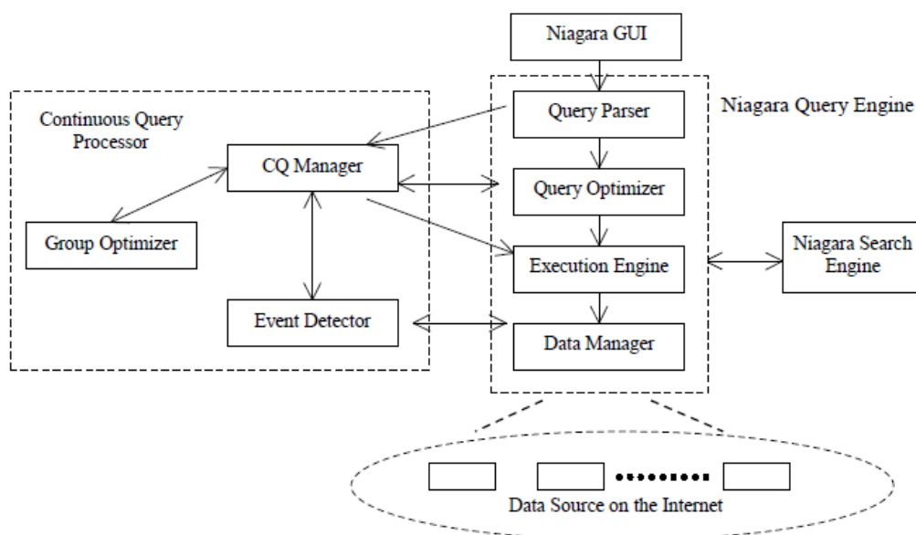
Figura 4.1. Arquitectura del sistema NiagaraCQ. Extraída de [3]
