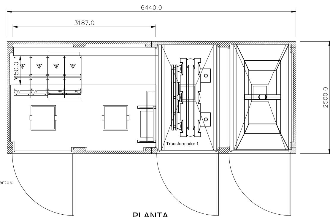
PLANTA
