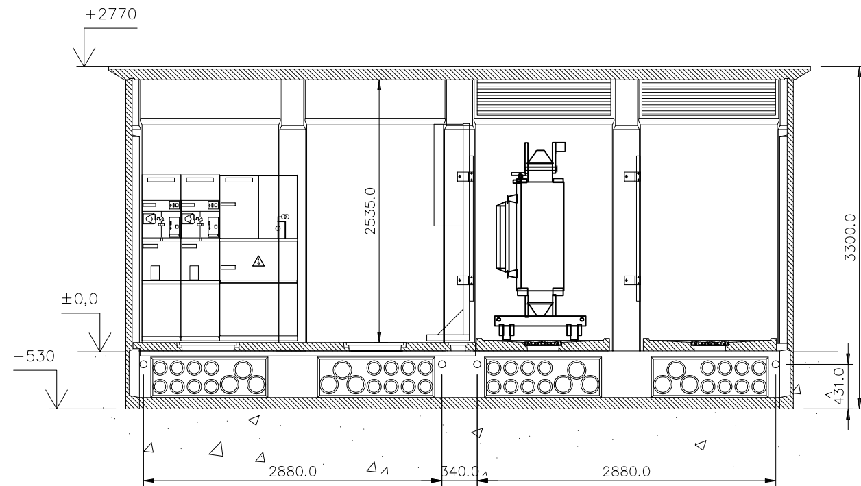
SECCIÓN
