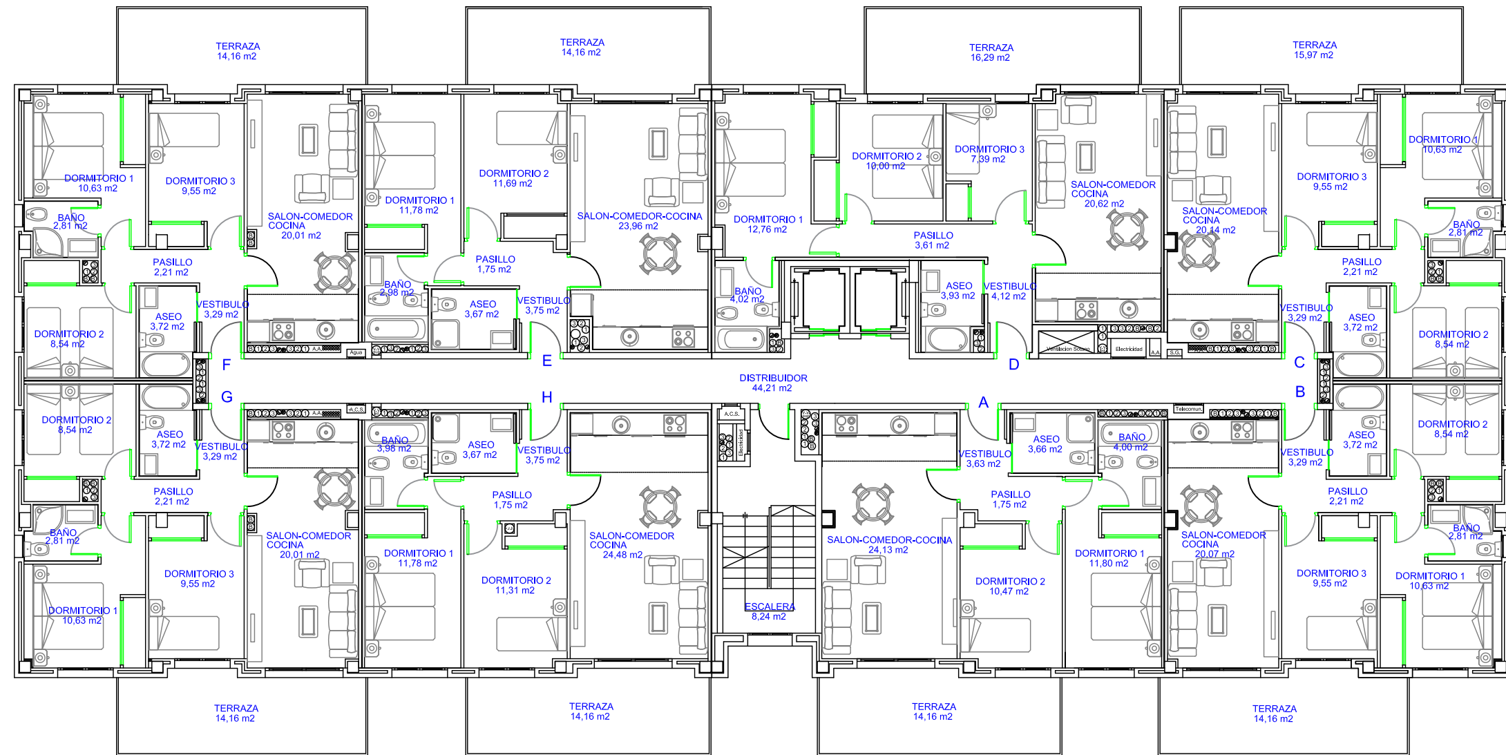
PLANTA TIPO (1ª, 2ª y 3ª) - DISTRIBUCIÓN Y SUPERFICIES
