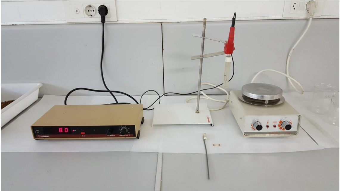
Ilustración 16. Instrumentos utilizados para la medición del pH.
