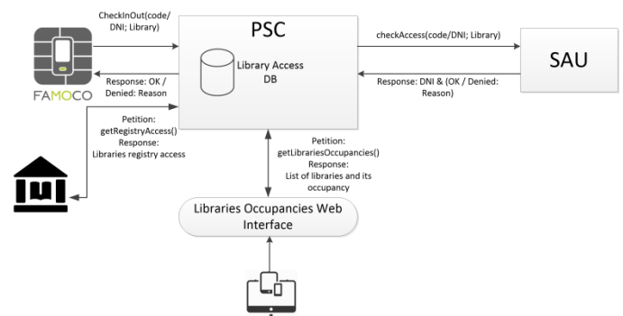
Figura 1. Arquitectura caso de uso de la biblioteca
