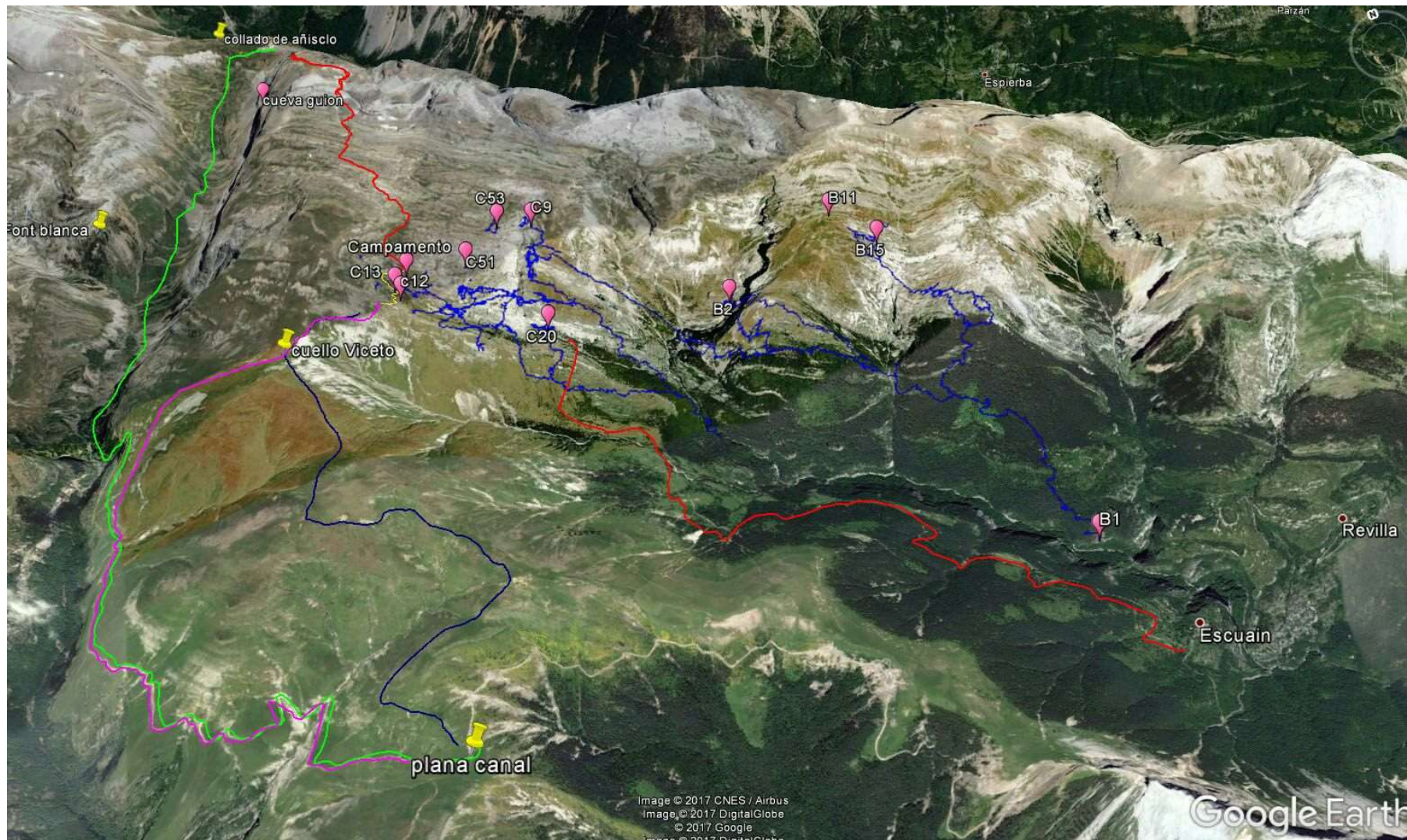
Modelo en 3D de la zona de estudio. En azul, se localiza el Sistema Fuentes de Escuaín. También con un marcador de color rosa se sitúan las correspondientes bocas de entrada a la caverna.
