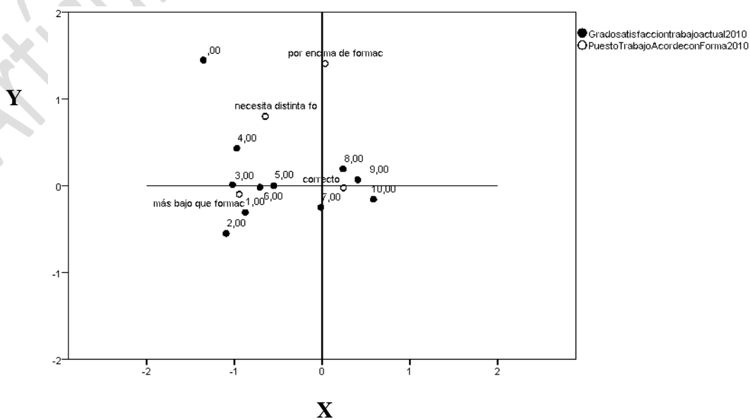
Fig. 2. Representación gráfica de los puntos de fila y de columna. Normalización simétrica
