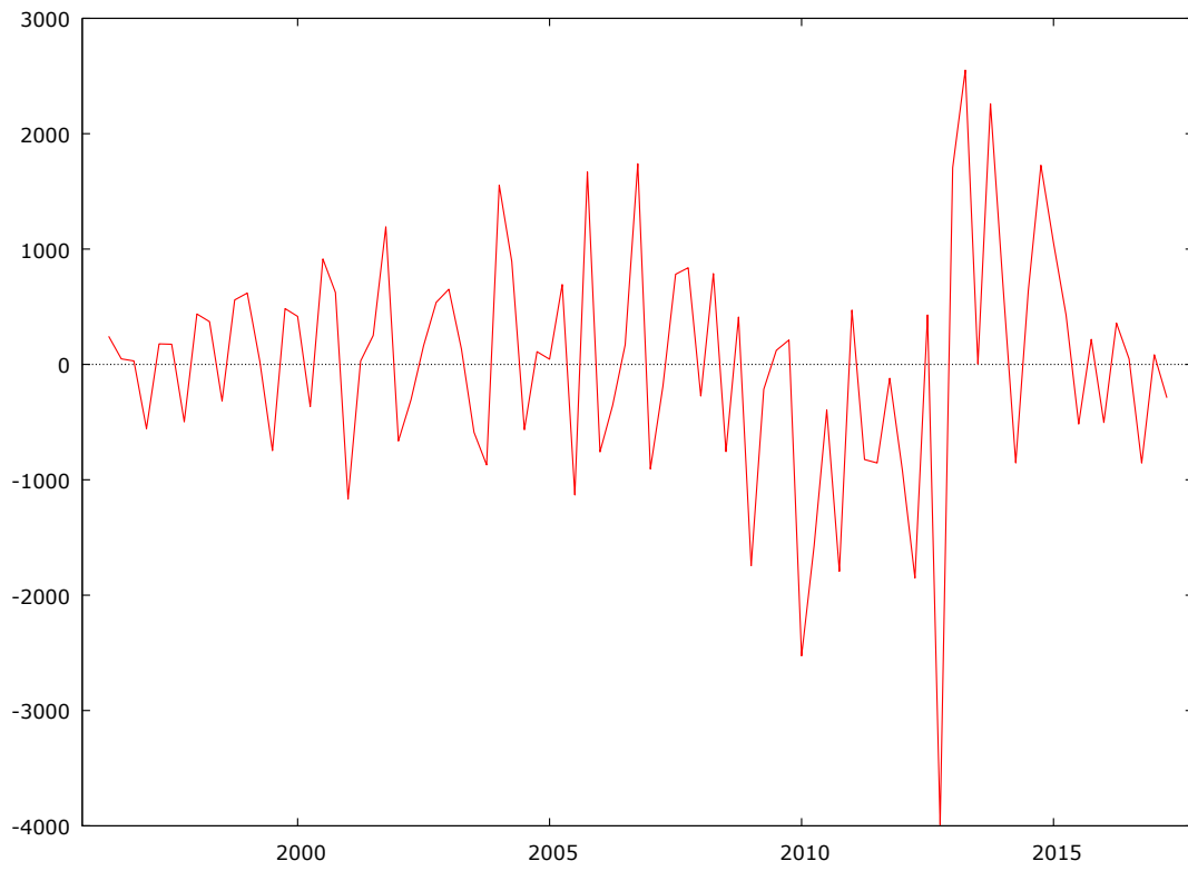
Residuos de la regresión (= CFAAPP observada - estimada)
