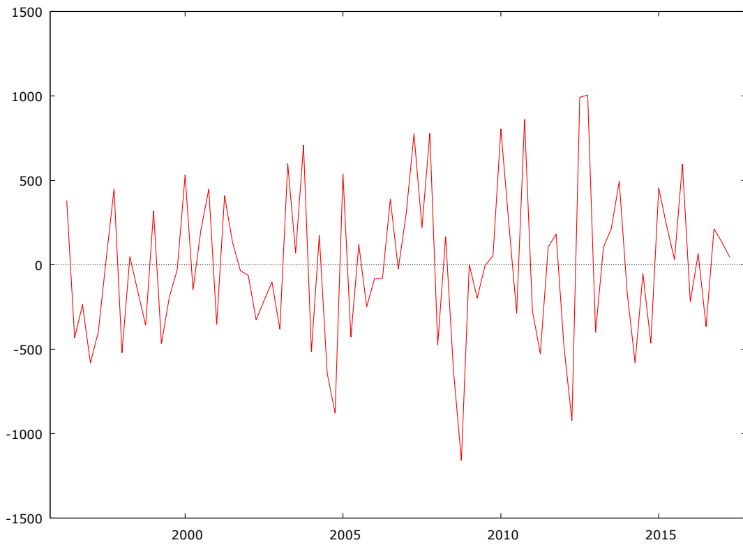
Residuos de la regresión (= AGR observada - estimada)
