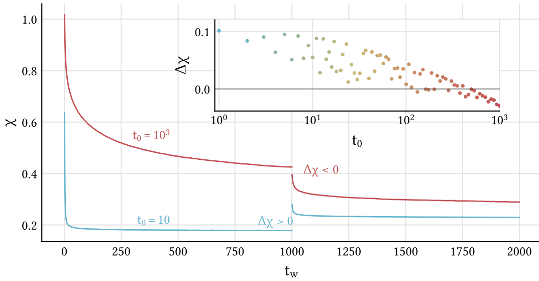
Figura 4.1: Susceptibilidad \chi para T_1 = 0.9, T_2 = 0.5, L = 8 promediadas sobre 31500 muestras con valores de t_0 \in [1, 10^3] , color en el original. El rejuvenecimiento fuerte desaparece cuando t \approx \frac{1}{2}10^3 .
