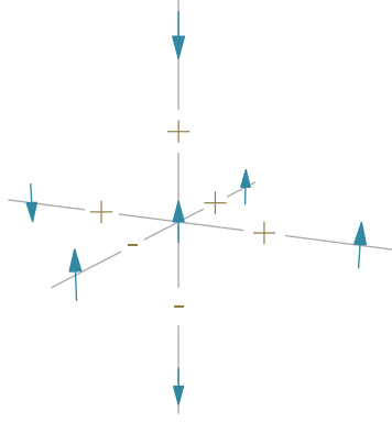
Figura 1.2: Modelo de Edwards-Anderson en 3D, con interacciones a primeros vecinos. Cada espín interactúa únicamente con los 6 espines más cercanos en la red, siendo el signo de la interacción aleatorio.
