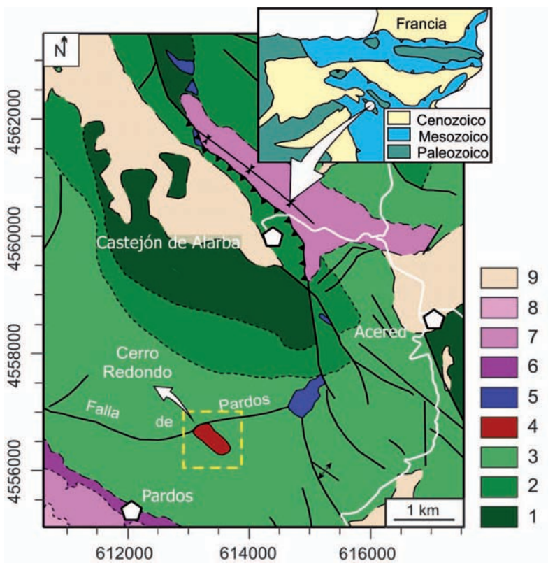
Fig. 1.- Mapa geológico de situación del magmatismo de la Sierra de Pardos. 1: Cámbrico Medio-Superior, 2: Cámbrico-Ordovícico Inferior, 3: Ordovícico Inferior, 4: Dacitas de Cerro Redondo, 5: Riolitas, 6: Facies Buntsandstein, 7: Facies Muschelkalk, 8: Facies Keuper, y 9: Cuaternario. Modificado de Gabaldón et al. (1980a y b). Ver figura en color en la Web.
