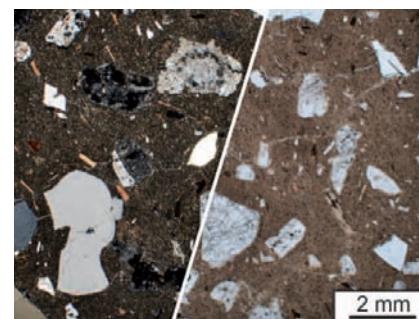
Fig. 2.-Aspecto al microscopio de las dacitas subvolcánicas en nicoles cruzados (izquierda) y paralelos (derecha). Ver figura en color en la Web.
