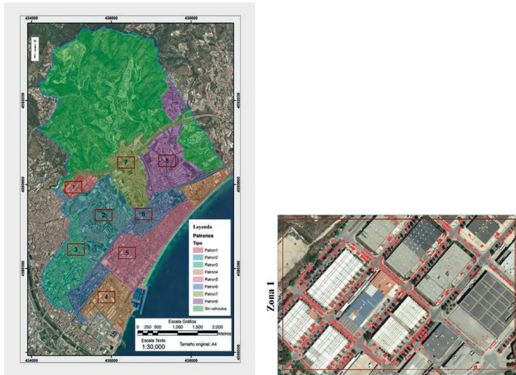
Figura 4 | Localización de las ocho zonas de análisis, patrones de ocupación vehicular y detalle de la delimitación de vehículos en la zona 1.
