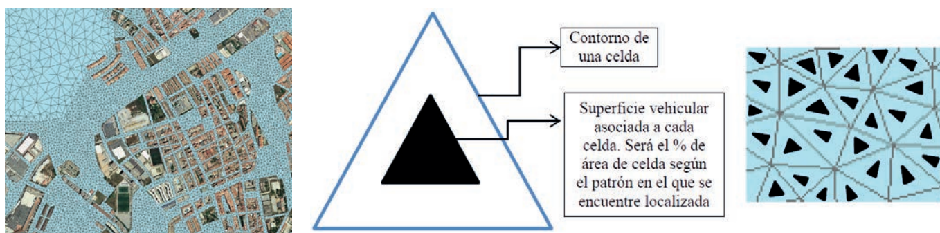
Figura 5 | Superficie vehicular asociada a una celda para la aplicación del método distribuido.
