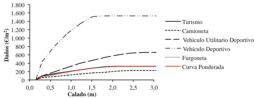
Figura 6 | Adaptación de las curvas del USACE y curva ponderada propuesta.
