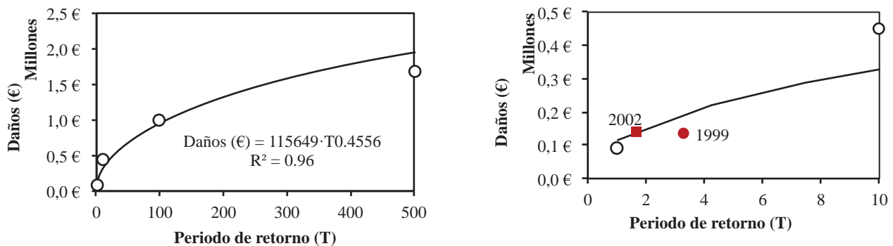
Figura 9 | Daños a vehículos en relación con el período de retorno de la lluvia de diseño, curva potencial de ajuste y representación de los eventos reales considerados para la validación del método.
