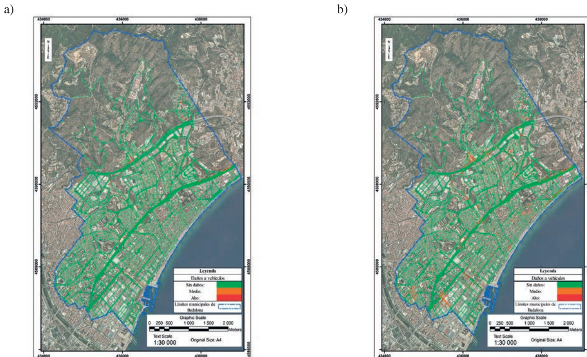
Figura 7 | Mapas de daños a vehículos para periodos de retorno de a) 10 y b) 500 años.
