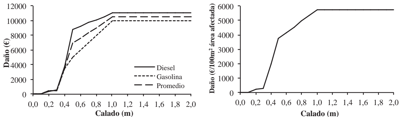
Figura 2 | Curvas de daños para las dos clases de vehículos considerados en el proyecto CRUE (izquierda) y curva adaptada a euros por 100 metros cuadrados de área afectada (derecha).
