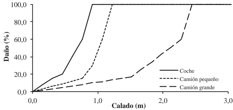
Figura 1 | Curvas de daños por tipo de vehículo propuestas en HAZUS-MH (FEMA).
