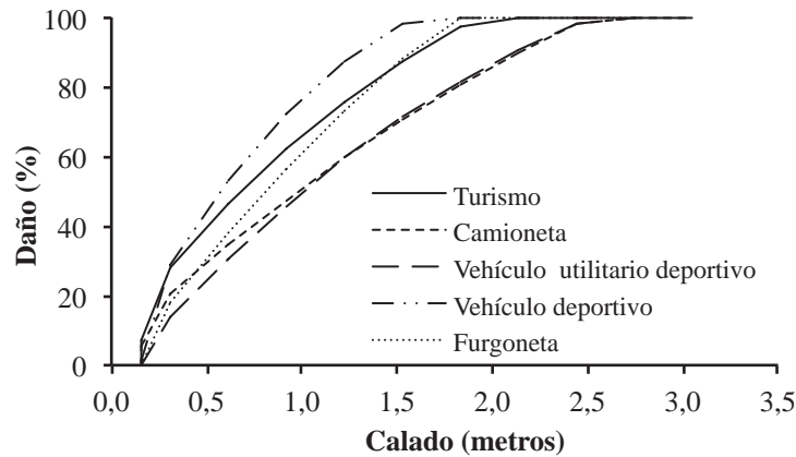
Figura 3 | Curvas de daños para vehículos desarrolladas por el USACE
