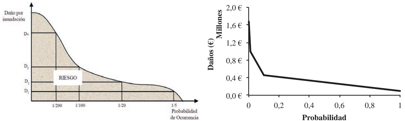
Figura 8 | Curva que relaciona el daño (expresado en €) con la probabilidad de ocurrencia (teórica a la izquierda y calculada a la derecha). El área bajo la curva representa el DAE.
