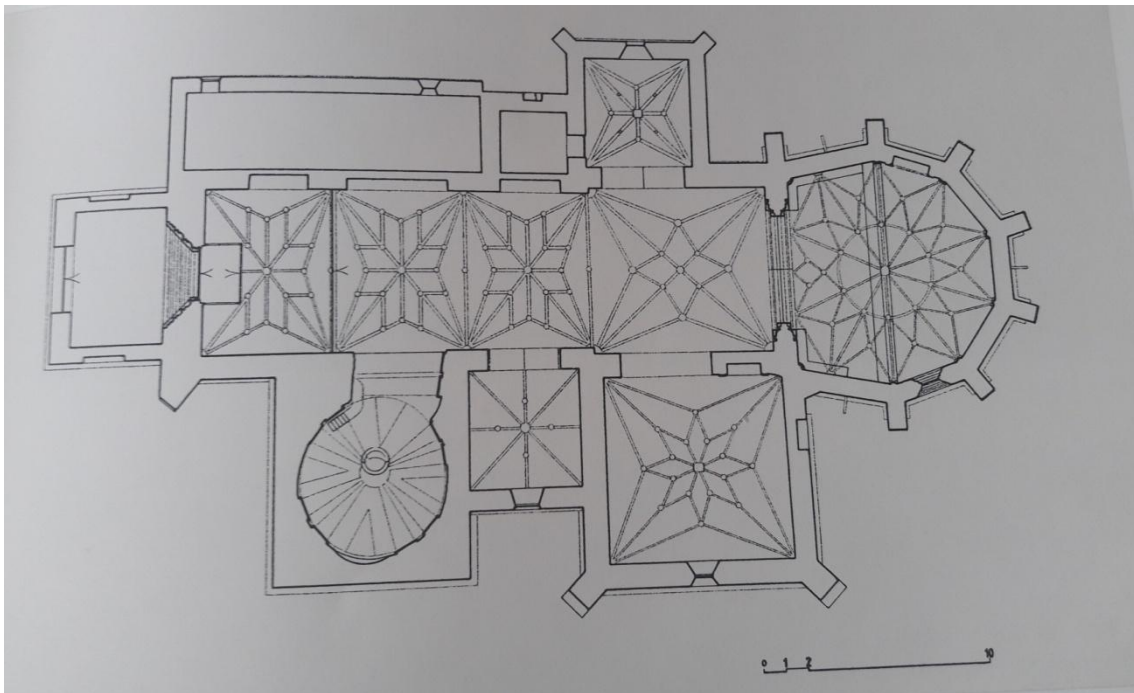
Ilustración 33: Iglesia de San Miguel Arcángel. Planta.
