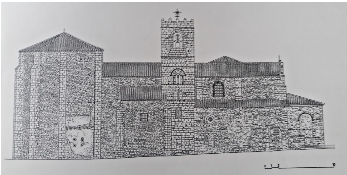
Ilustración 34: Iglesia de San Miguel Arcángel. Alzado norte.
