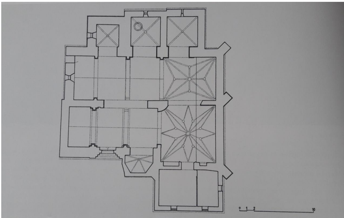
Ilustración 16: Iglesia de Ntra. Sra. de la Peña. Planta.
