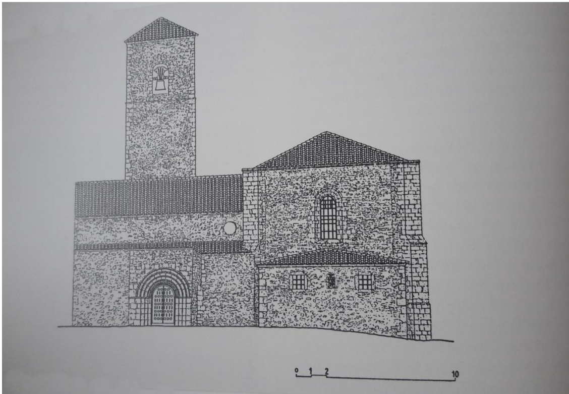
Ilustración 17: Iglesia de Ntra. Sra. de la Peña. Alzado Sur.
