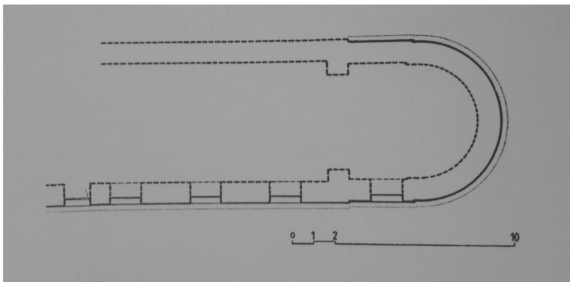
Ilustración 46: Sinagoga. Planta, antes de la última restauración.
