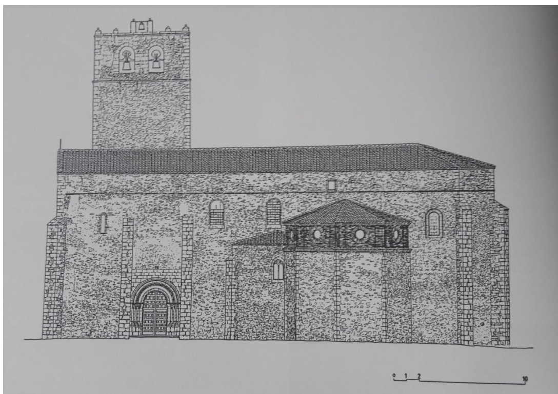
Ilustración 43: Iglesia de San Juan Bautista. Alzado sur.
