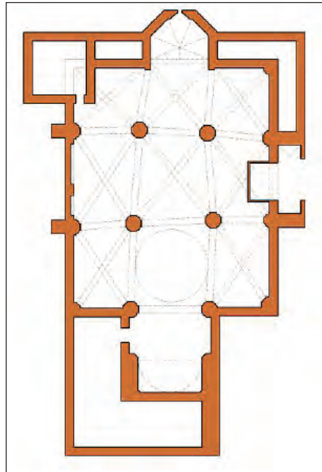
Fig. 7. Croquis de la planta de la iglesia de Santo Domingo de Silos de Daroca (Zaragoza) (José Ángel Gil Bordás).
