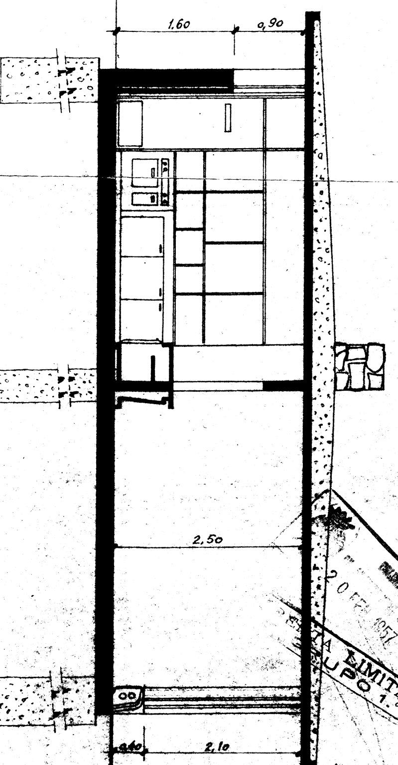
SECCION B-B
