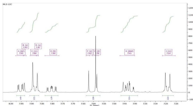
Figura 10. Espectro ^1\text{H} -RMN de CL-1d
