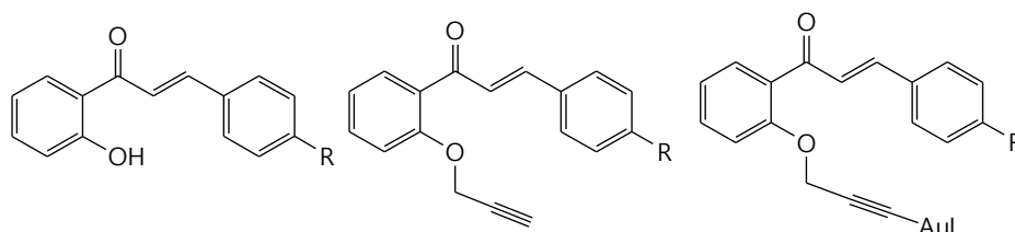
Figura 3. Estructura de 2-hidroxichalconas, chalconas alquiladas y complejos de oro con chalconas
