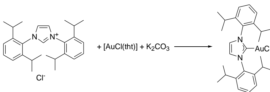
Ecuación 6. Síntesis del complejo [\text{ClAuIPr}]
