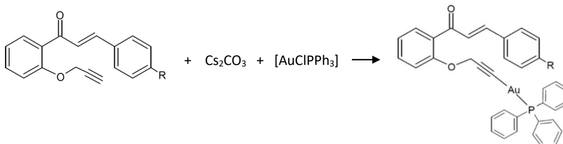
Ecuación 5. Síntesis de complejos con oro \text{PPh}_3
