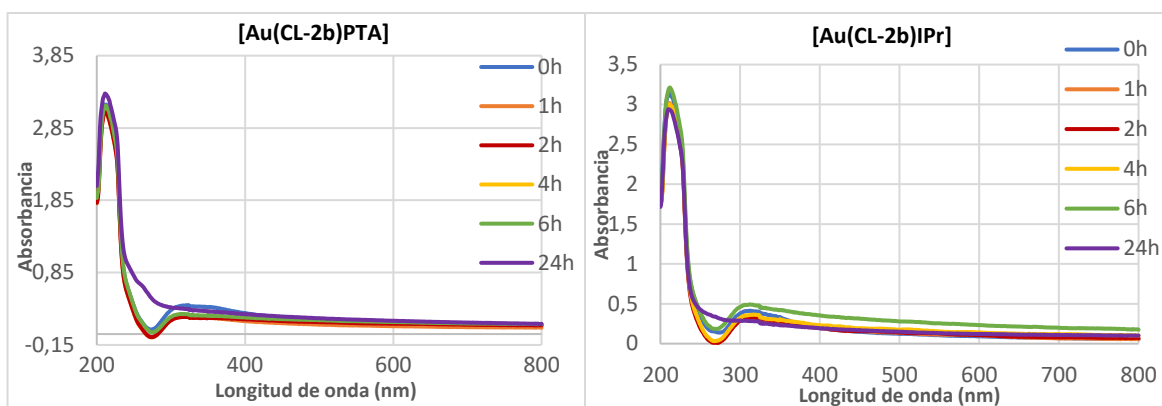
Figura 16. Espectro UV- Vis de [Au(CL-2b)PTA] (2) y [Au(CL-2b)IPr] (8) a lo largo del tiempo
