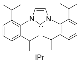
Figura 5. 1,3-bis(2,6-di- i -propilfenil)imidazol-2-ilideno (IPr)
