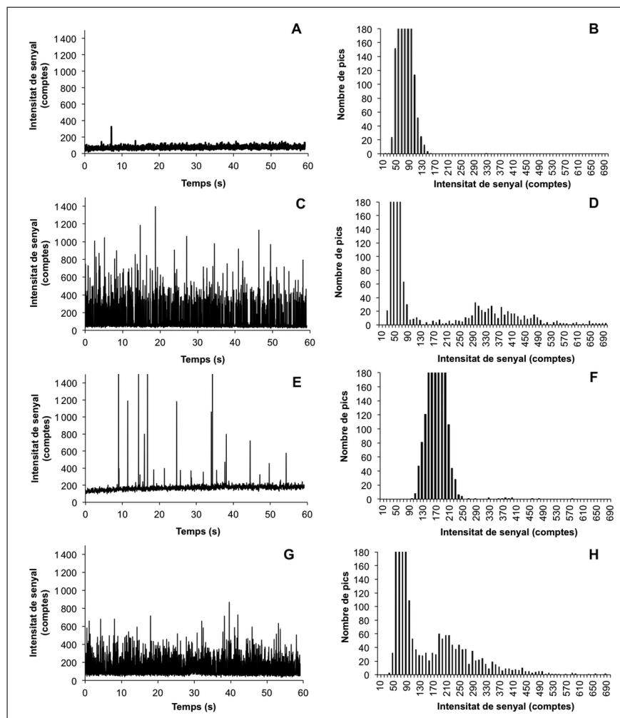
FIGURA 3. Representacions de la intensitat de senyal versus el temps i histogrames de l'anàlisi per SP-ICP-MS dels lixivats dels sòls contaminats amb AgNP-citrat de 40 nm (A, B), AgNP-citrat de 100 nm (C, D), AgNP-PEG de 100 nm (E, F) i AgNP-PVP de 100 nm (G, H).
