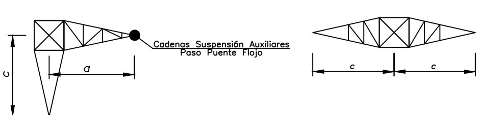
VISTA A-A'
