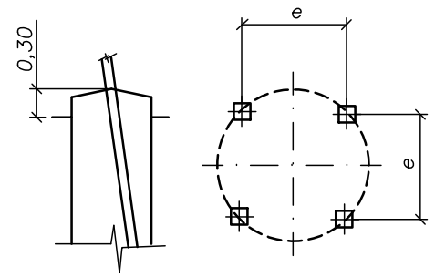
DETALLE A
