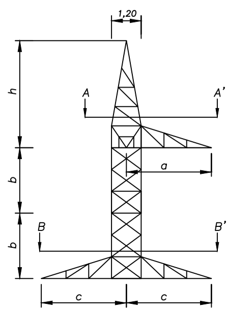
ARMADOS APOYOS T-01 Y T-45
