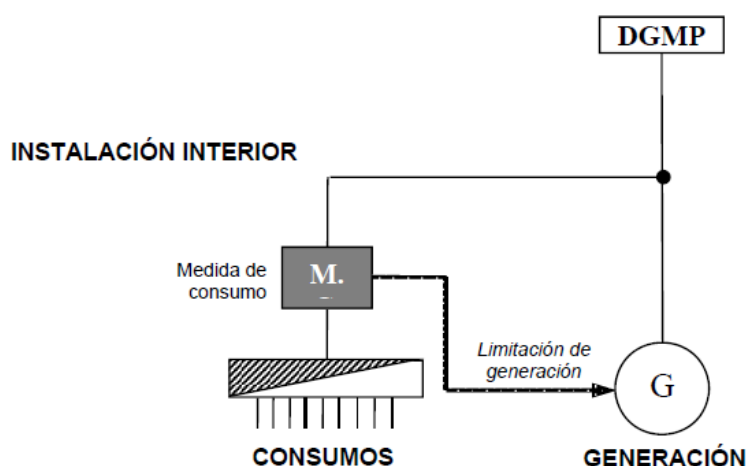
Figura 5 - Esquema de instalación con generación fotovoltaica conectada a red (Fuente: Real Decreto 244/2019)
