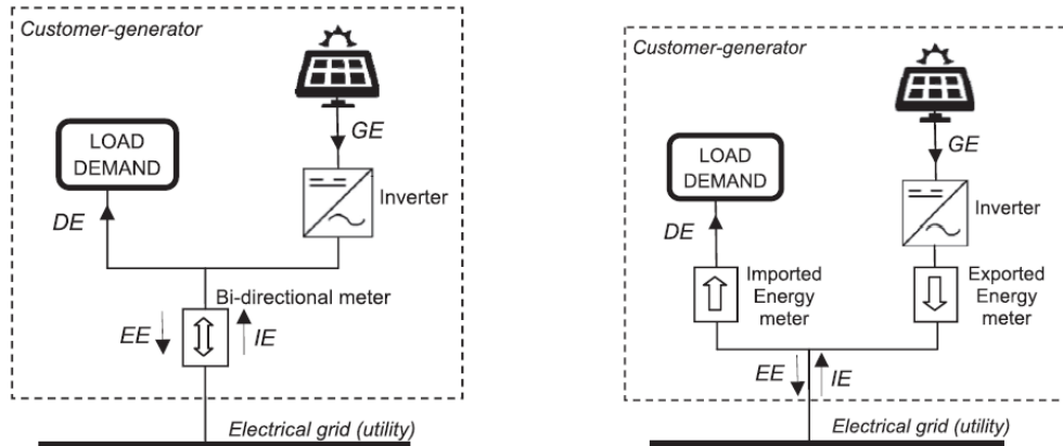
Figura 4 - Esquemas de instalaciones en las que se realiza Net metering (1) y Net billing (2) (Fuente: [31])
