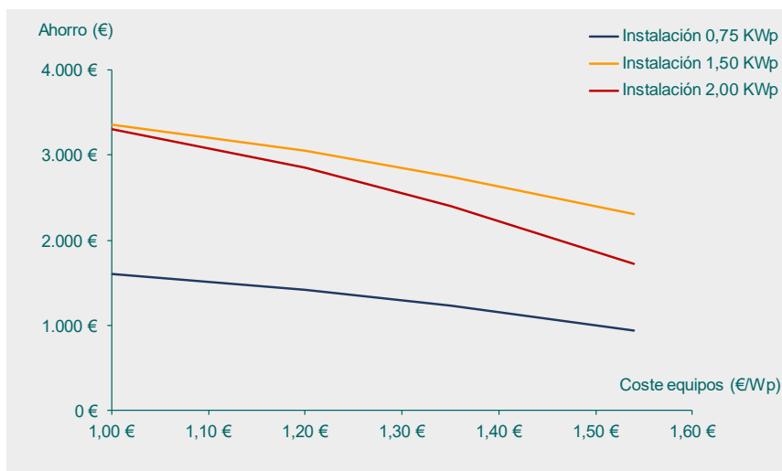
Figura 13 - Comparativa de ahorro (€) entre configuraciones con diferente potencia instalada y diferente coste de instalación de los equipos (€/Wp)
