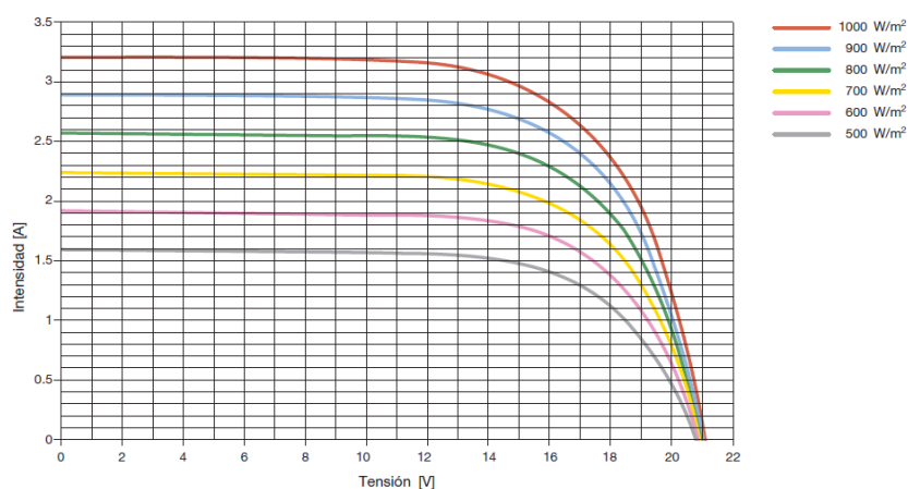
Figura 7 - Curva I-V de un panel fotovoltaico estándar (fuente: ABB)
