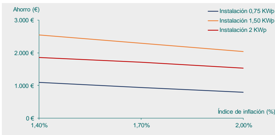
Figura 15 - Comparativa de ahorro (€) entre configuraciones con diferente potencia instalada y diferente índice de inflación (%)
