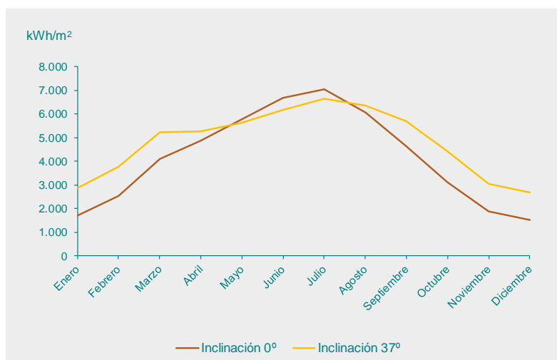
Figura 8 - Curvas de irradiancia media diaria para inclinaciones de 0° y 37°
