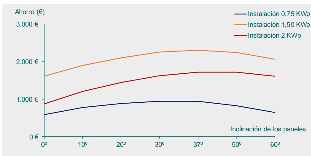
Figura 17 - Comparativa de ahorro (€) entre configuraciones con diferente potencia instalada y diferentes ángulos de inclinación de los paneles
