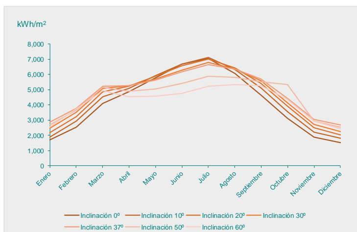
Figura 16 - Curvas de irradiancia para diferentes ángulos de inclinación de los paneles
