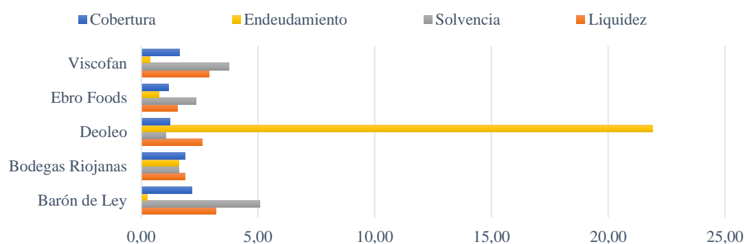
Figura 3.3: Relaciones lógicas
