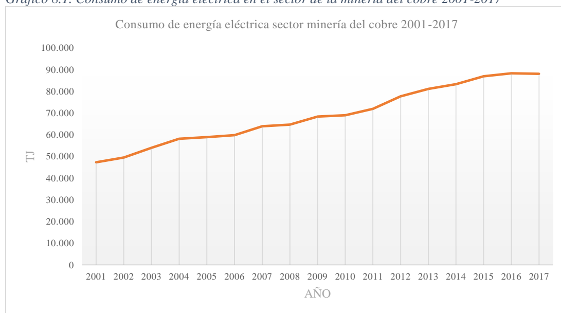
Gráfico 8.1. Consumo de energía eléctrica en el sector de la minería del cobre 2001-2017
