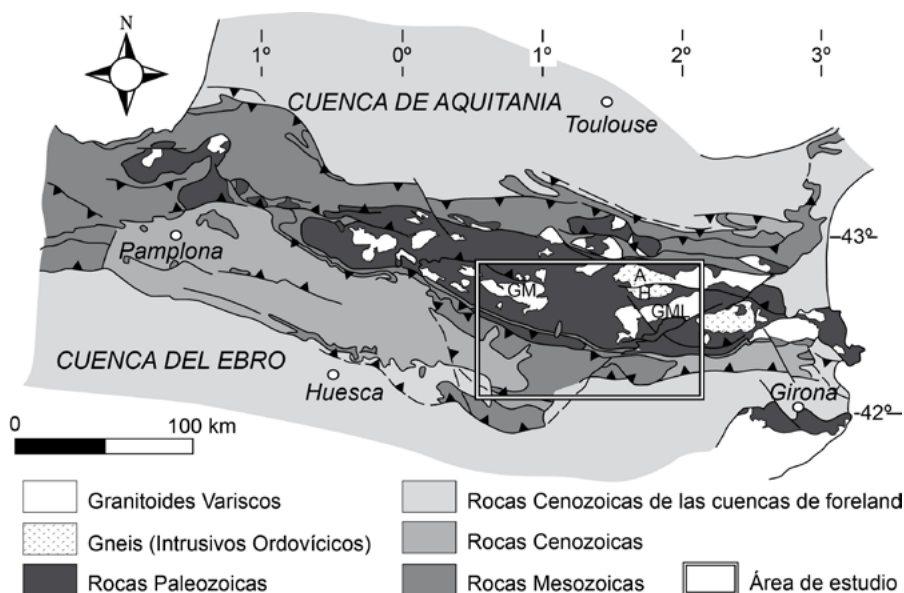
Fig. 1.- Esquema geológico de los Pirineos. La zona de estudio está marcada con el recuadro. Ver figura en color en la web.
