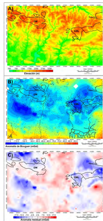
Fig. 2.- A) Modelo digital del terreno de la zona de estudio con la localización de las 824 nuevas estaciones. B) Anomalía de Bouguer con todas las estaciones utilizadas para su cálculo (3714). C) Anomalía de Bouguer residual. Los mapas muestran los contornos de los granitos objeto de estudio (GM: granito de La Maladeta; GML: granito de Andorra-Mount Louis). Ver figura en color en la web.
