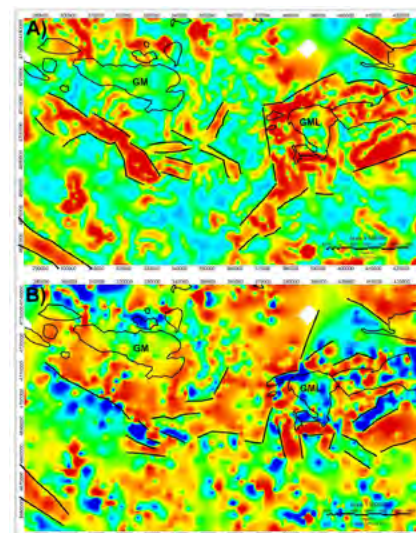
Fig. 3.- A) Derivada horizontal de la anomalía de Bouguer con los lineamientos más relevantes. B) Derivada vertical de la anomalía de Bouguer con los lineamientos más relevantes. Los mapas muestran los contornos de los granitos objeto de estudio. Ver figura en color en la web.
