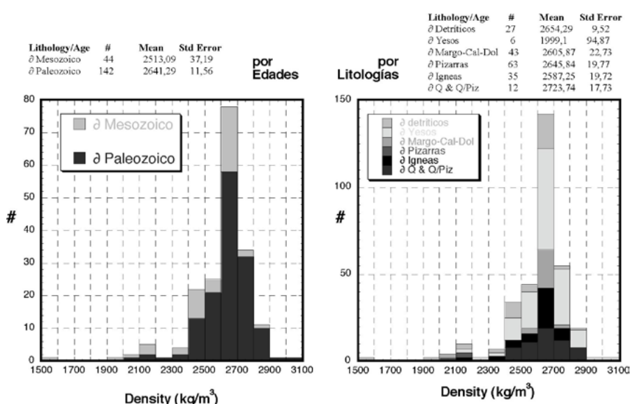
Fig. 4.- Histogramas de densidad por edades y por litologías de las 186 muestras analizadas. Fig. 4.- Age and lithology density histograms of the 186 samples analyzed.
