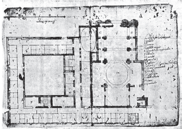
Figura 23. Antonio FORCADA, planta del colegio de la Compañía de Jesús de Calatayud, antes de 1745. Extraída de Guillermo FURLONG, «Algunos planos de Iglesias y Colegios de la Compañía de Jesús en España», Archivum Historicum Societatis Iesu , XXVIII, 55 (Roma, 1959), plano n.º 9.
