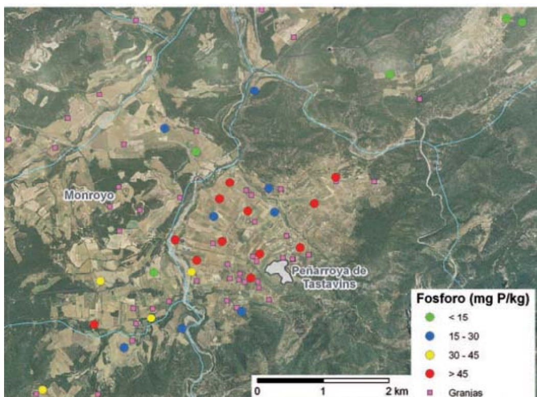
Figura 11.- Resultados de fósforo en la 4ª campaña de muestreo de Peñarroya de Tastavins
