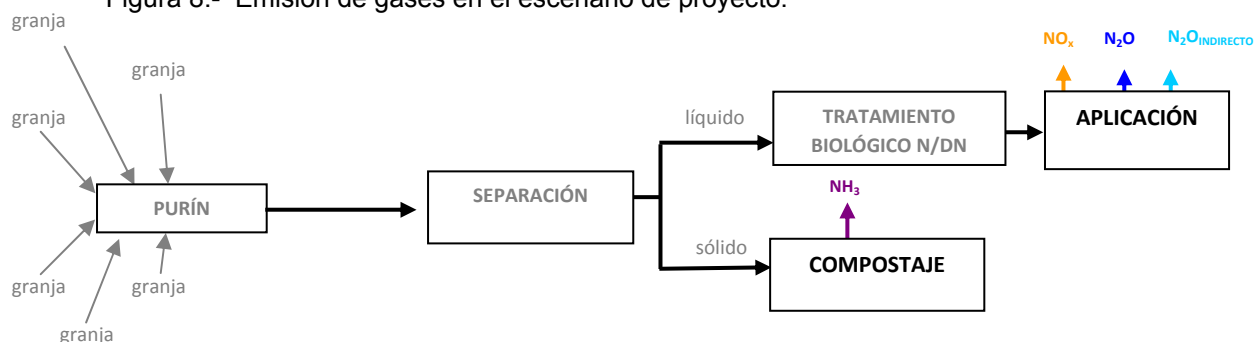
Figura 8.- Emisión de gases en el escenario de proyecto.
