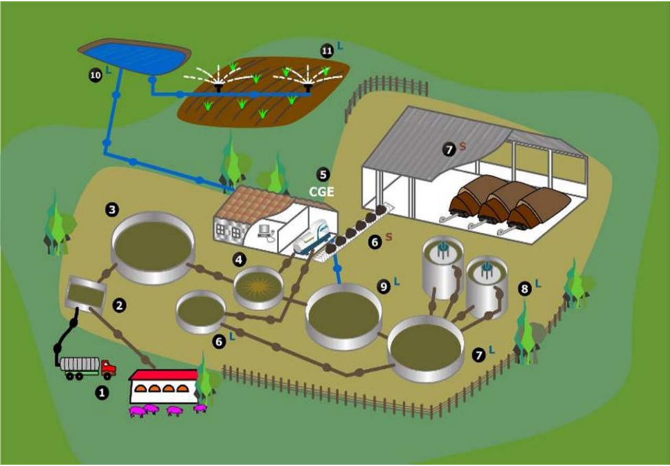
Figura 3.- Esquema de planta de tratamiento.
