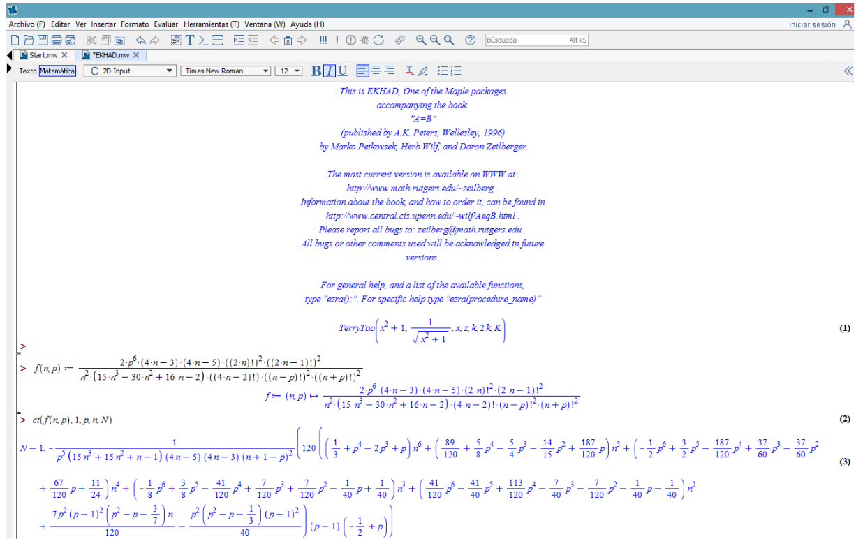
Figura 3.2: Demostración con Maple y EKHAD de (iii)
