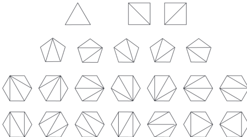
Figura 1.1: Polígonos triangulados
