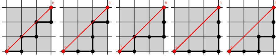
Figura 1.6: Solución para n = 3 .
