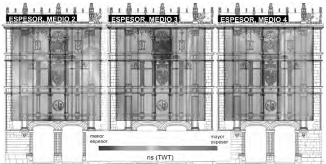
Fig. 4.- Resultados obtenidos de la correlación lateral de variaciones del espesor de las unidades identificadas en los perfiles de georradar. Ver figura en color en la web.
