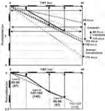
Fig. 3.- a) Evaluación de velocidades para distintos medios naturales y profundidades. b) Análisis de los espesores de distintas unidades comparadas con los sondeos realizados en la zona y cálculo de velocidades medias para los distintos medios existentes en la zona. Ver figura en color en la web.
